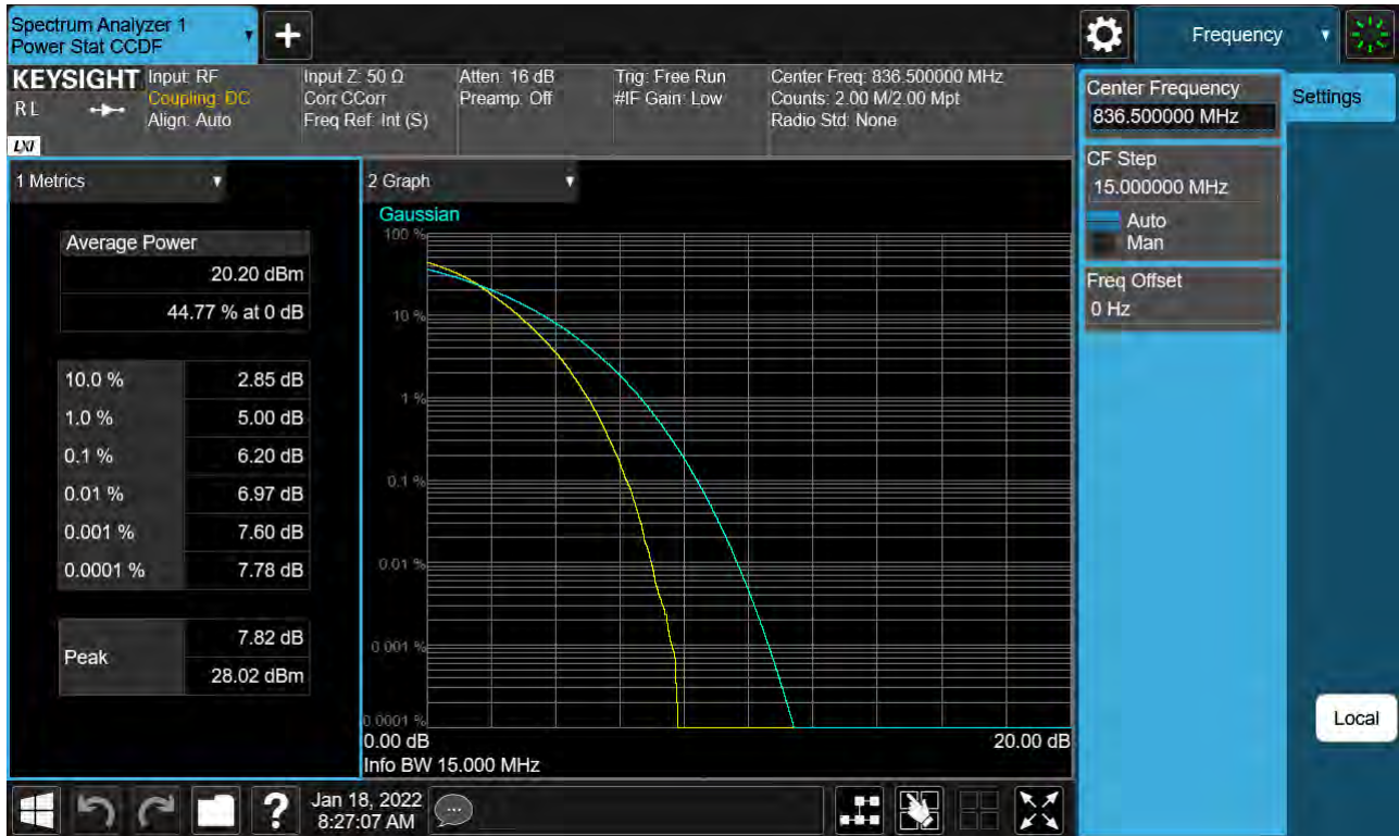
Sub6 n5. PAR Plot (15 M BW_Ch. 167300_256QAM_Full RB_0)
