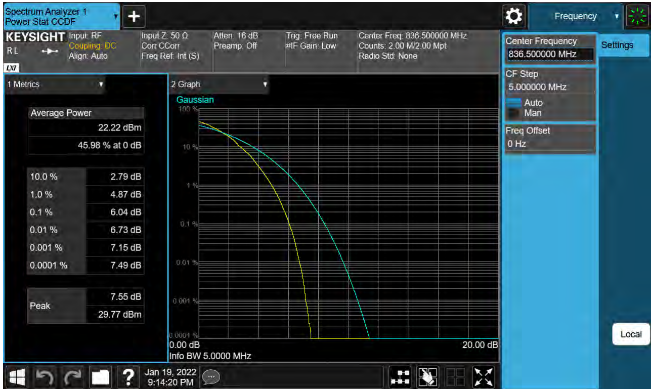
Sub6 n5. PAR Plot (5 M BW_Ch. 167300_64QAM_Full RB _0)
