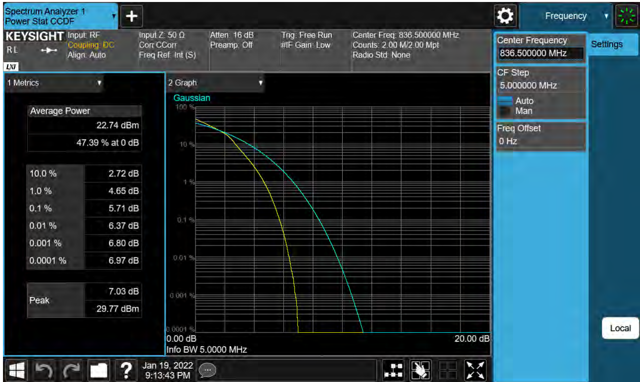
Sub6 n5. PAR Plot (5 M BW_Ch. 167300_16QAM_Full RB _0)
