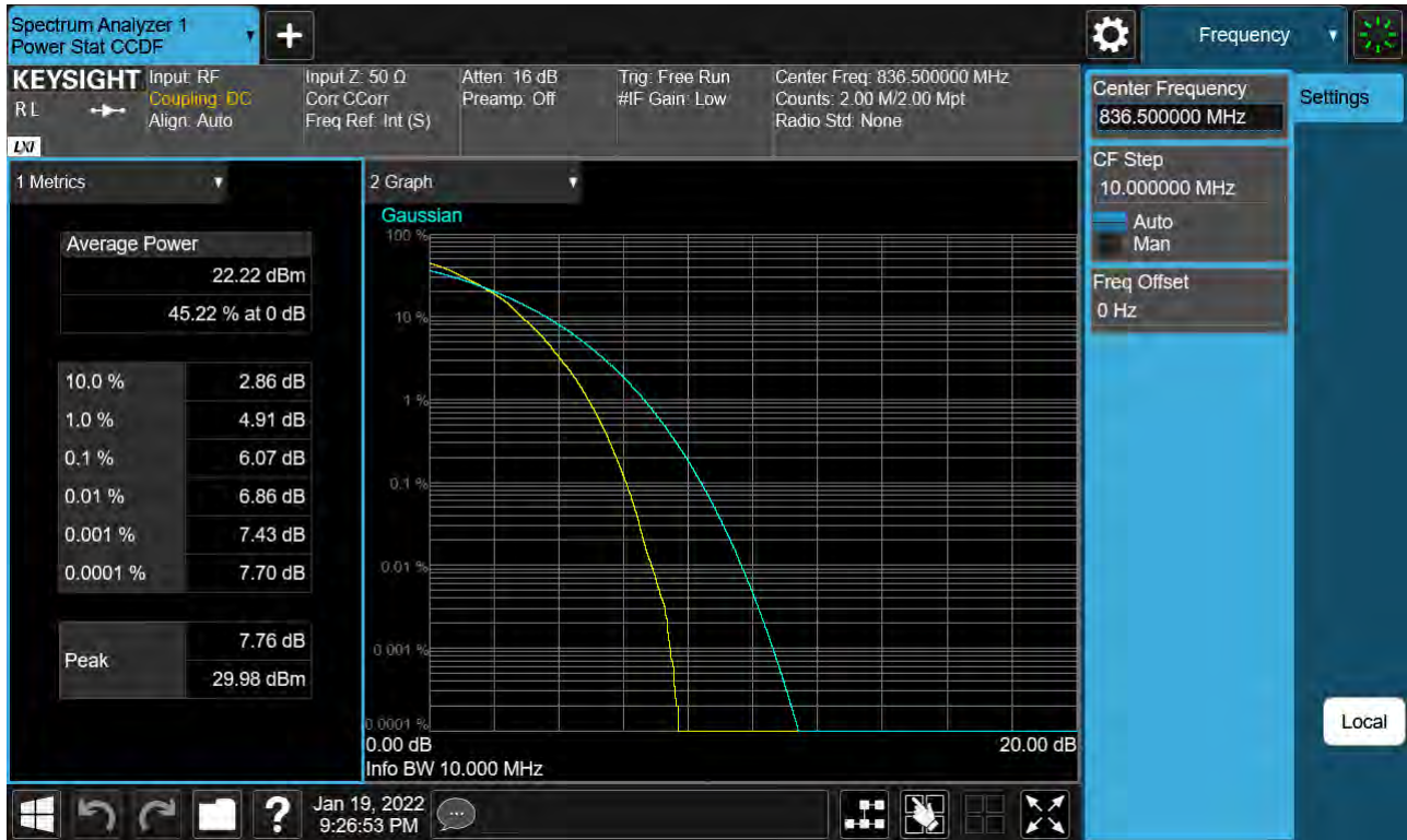
Sub6 n5. PAR Plot (10 M BW_Ch. 167300_64QAM_Full RB _0)
