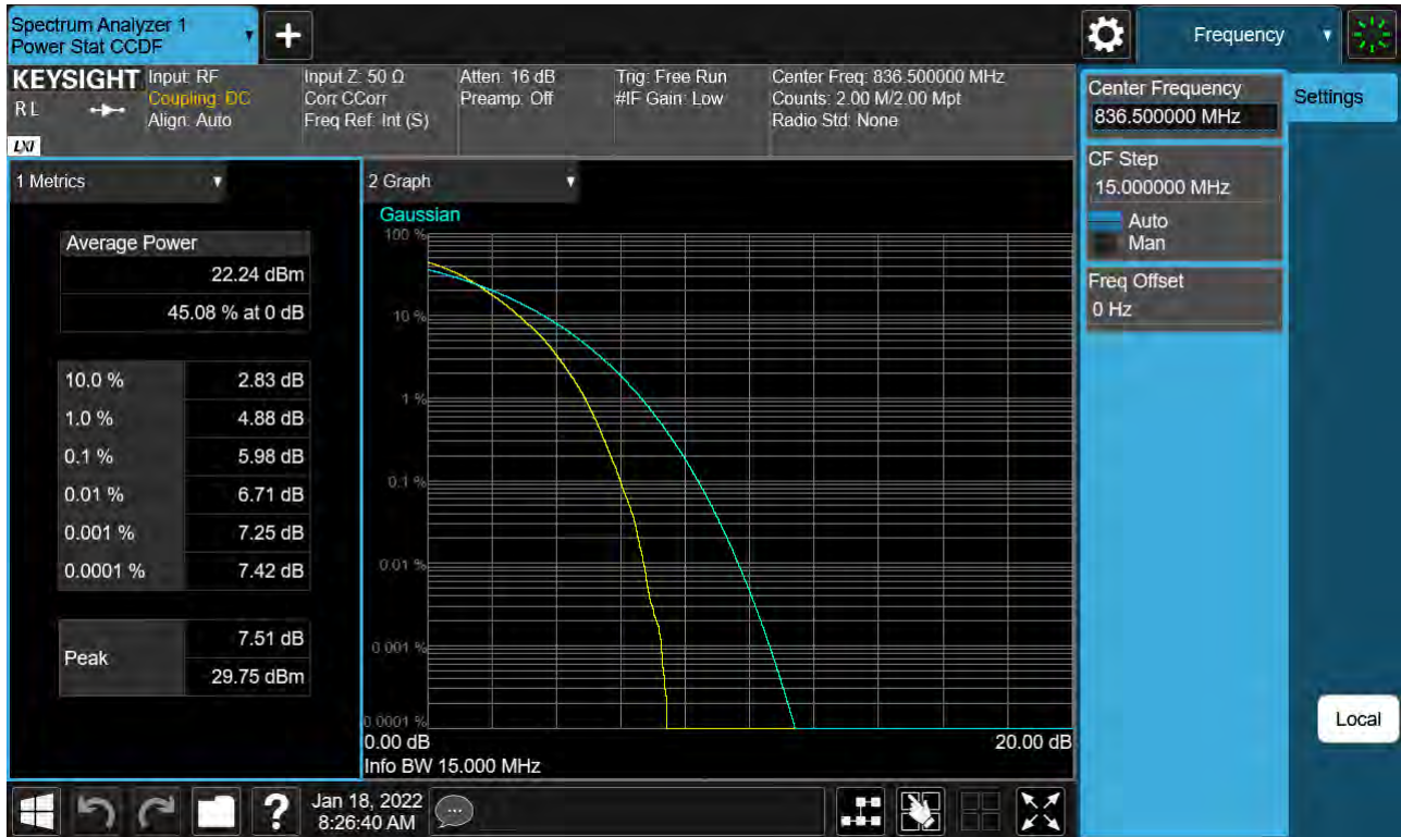
Sub6 n5. PAR Plot (15 M BW_Ch. 167300_64QAM_Full RB _0)
