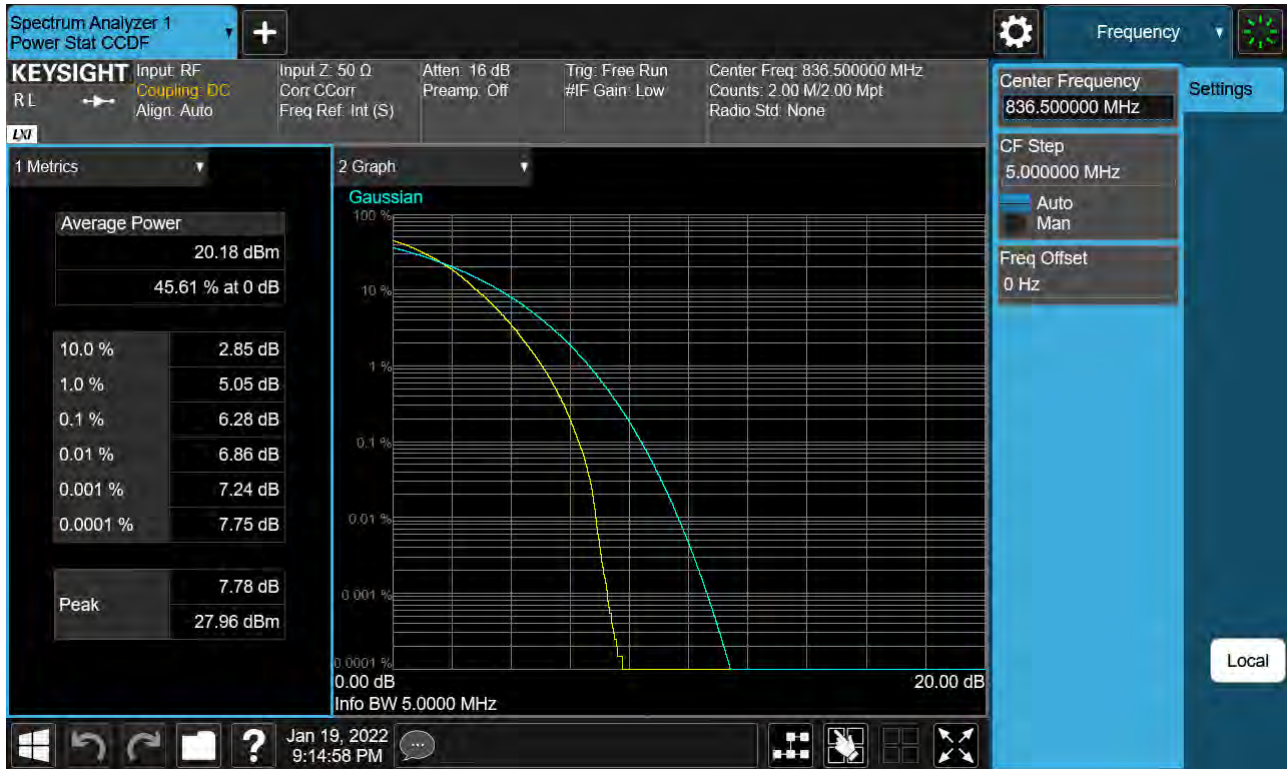
Sub6 n5. PAR Plot (5 M BW_Ch. 167300_256QAM_Full RB _0)
