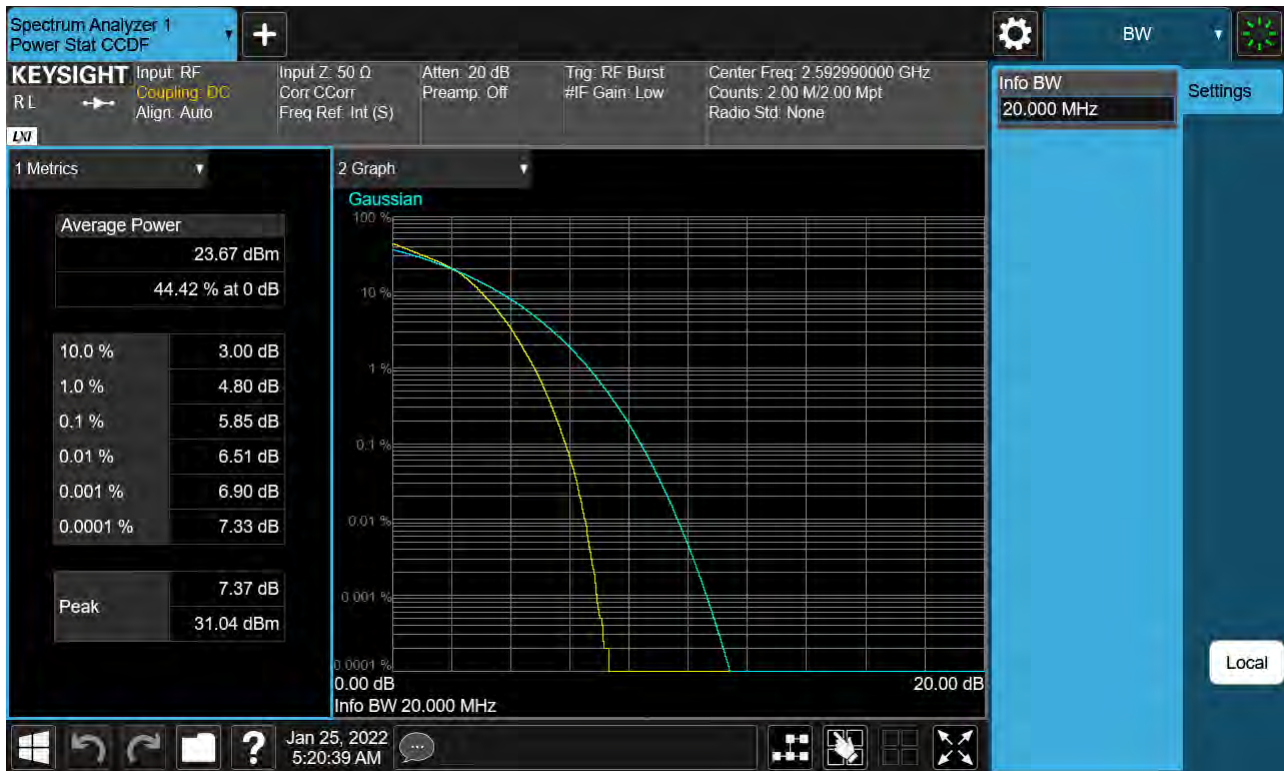
Sub6 n41. PAR Plot (20 M BW_Ch.518598_16QAM)
