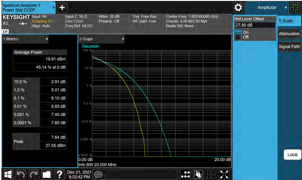
Sub6 n25(2). PAR Plot (20 M BW Ch.376500 256QAM _ Full RB _0)
