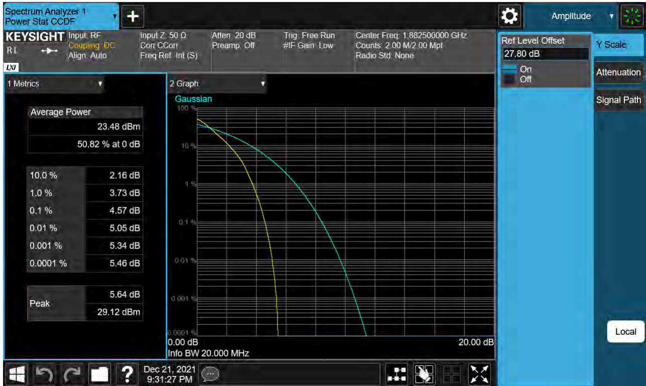
Sub6 n25(2). PAR Plot (20 M BW Ch.376500 QPSK _ Full RB _0)
