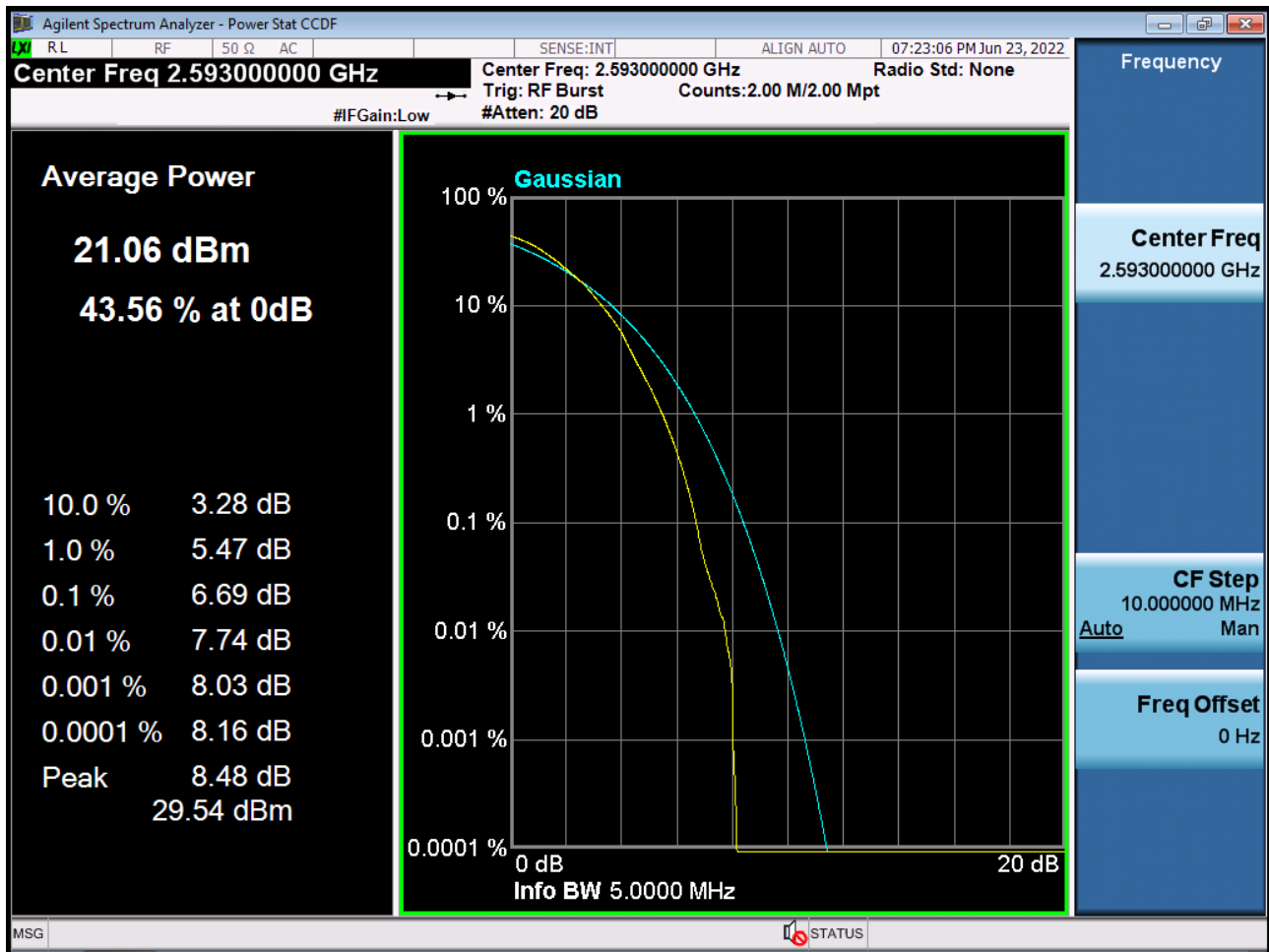
PAR Plot (5 M BW_Ch.40620_64QAM_RB25_0)
