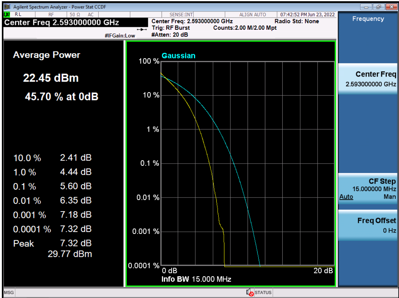
PAR Plot (15 M BW_Ch.40620_QPSK_RB75_0)
