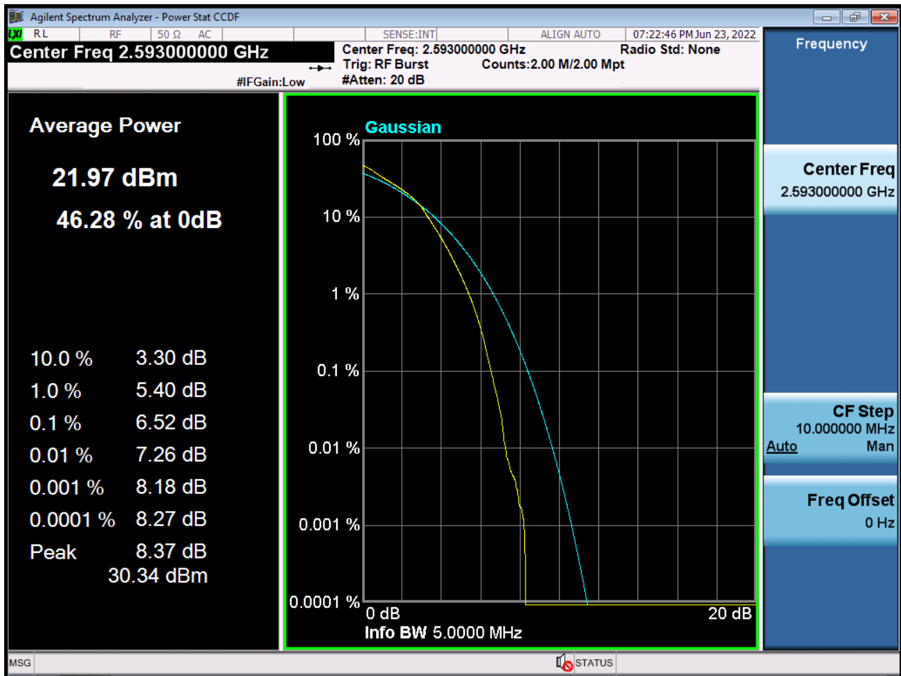
PAR Plot (5 M BW_Ch.40620_16QAM_RB25_0)
