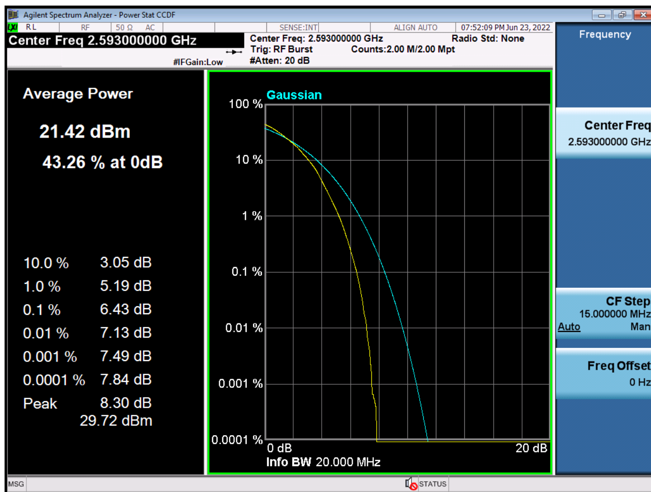
PAR Plot (20 M BW_Ch.40620_64QAM_RB100_0)
