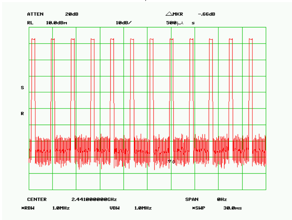
Bluetooth Mode, Basic Rate DH 1
