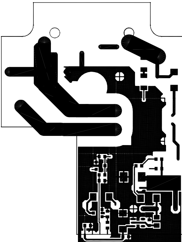
底层走线
