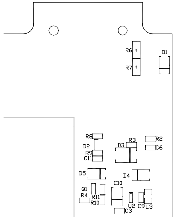
底层丝印
