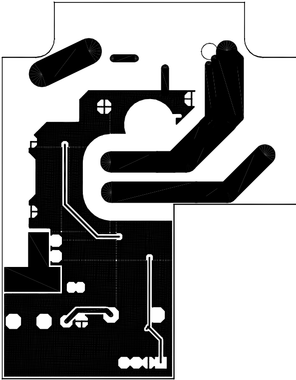
顶层走线
