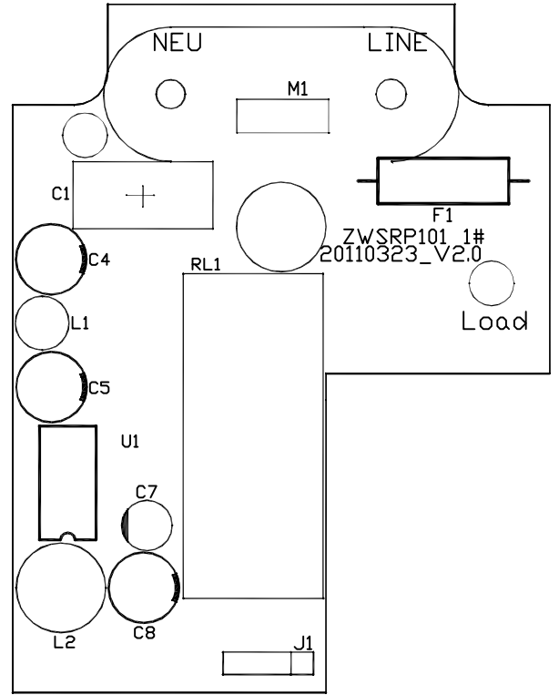
顶层丝印
