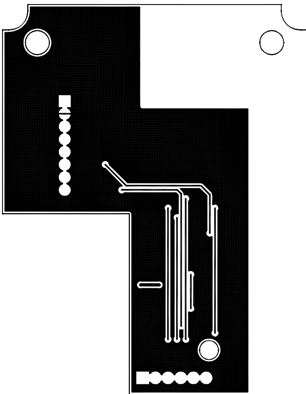
底层走线
