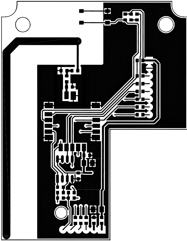
顶层走线
