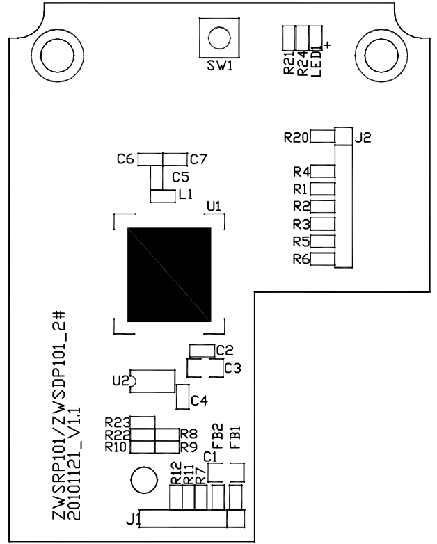
顶层丝印
