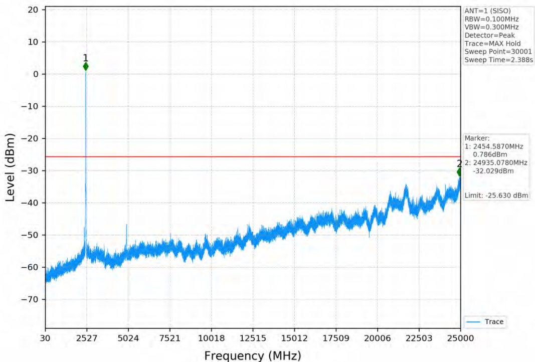
802.11n(HT20) SISO ANT1 REF
