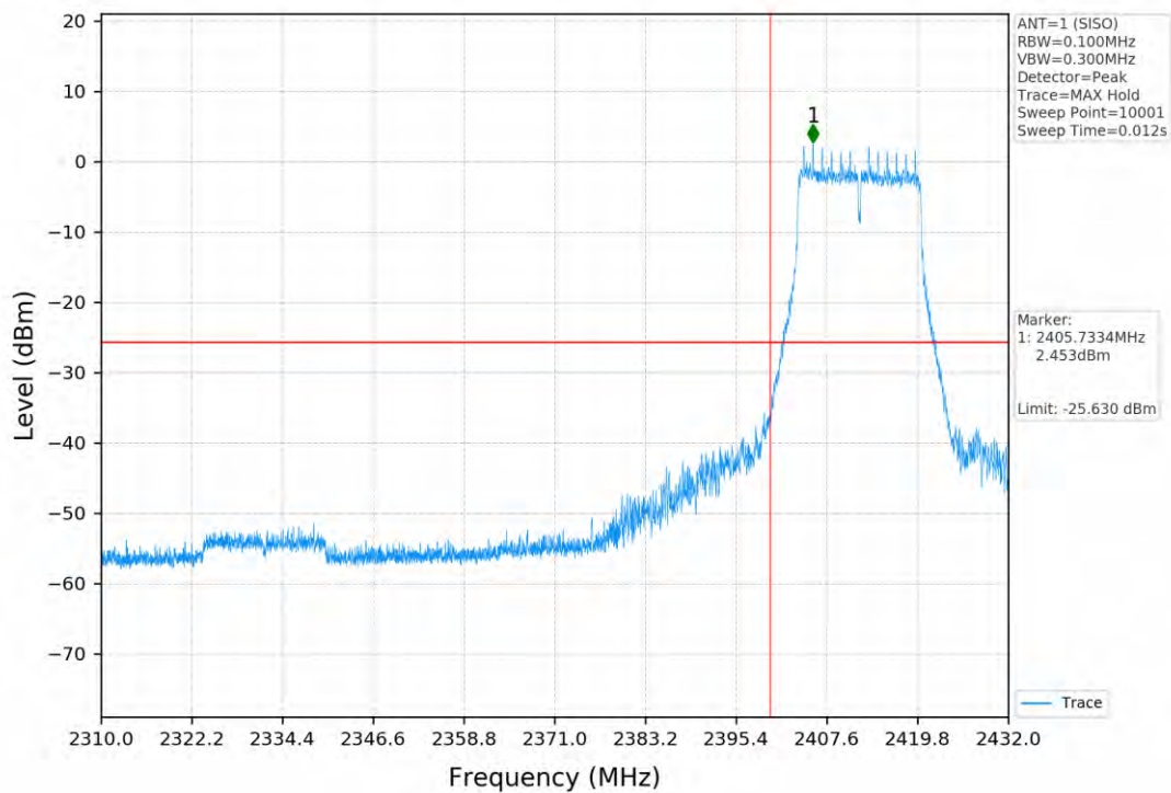
802.11g_2412MHz_SISO_ANT1
