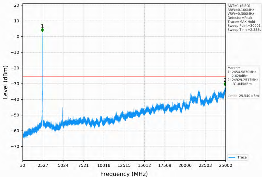
802.11n(HT40) SISO ANT1 REF
