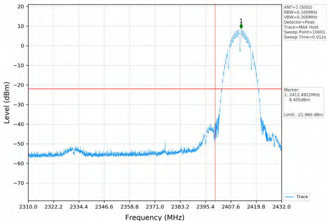
802.11b_2412MHz_SISO_ANT1
