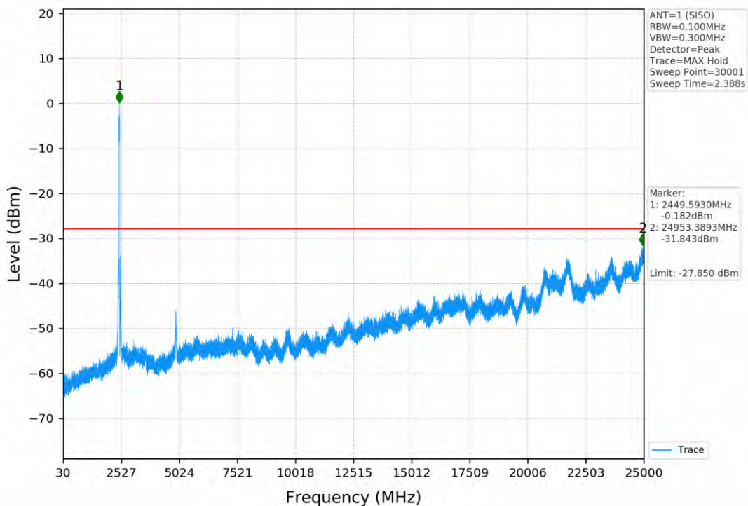
802.11n(HT40) 2452MHz SISO ANT1
