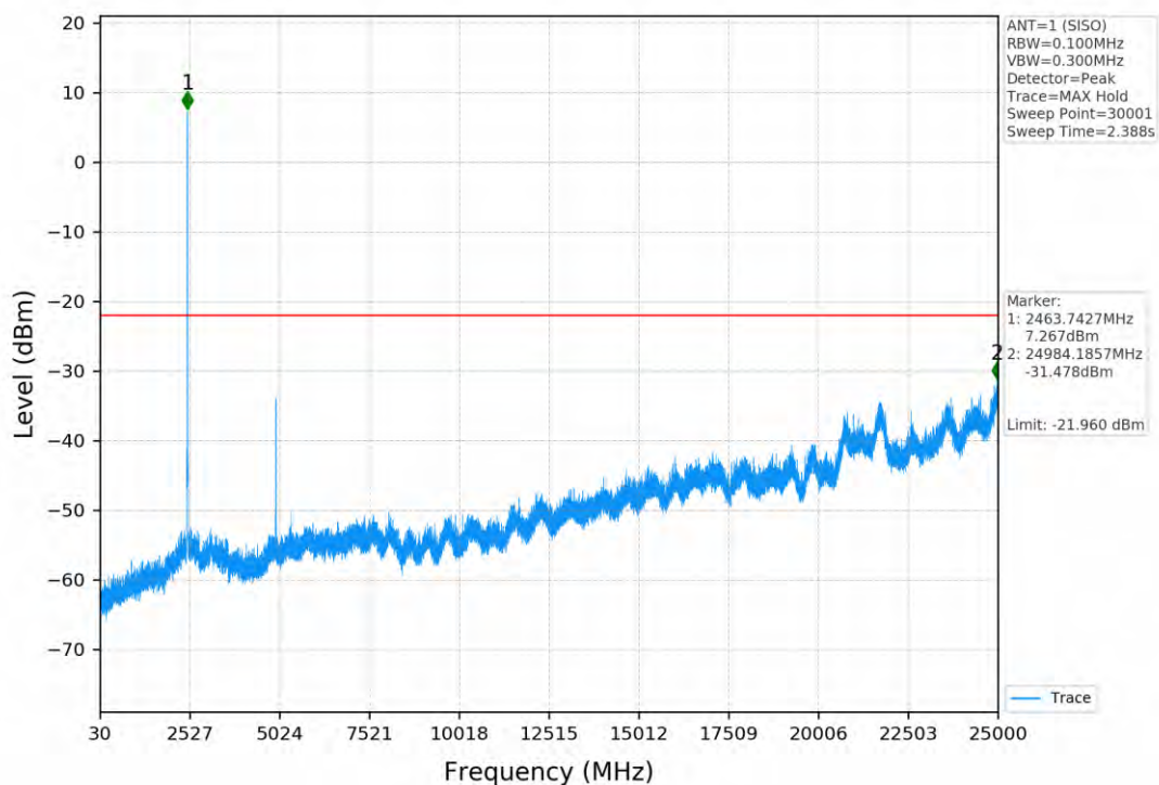
802.11g SISO ANT1 REF
