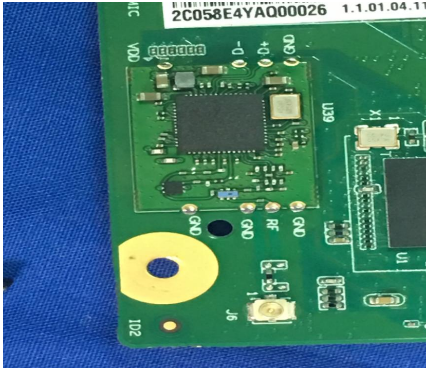
(6) EUT Photo
