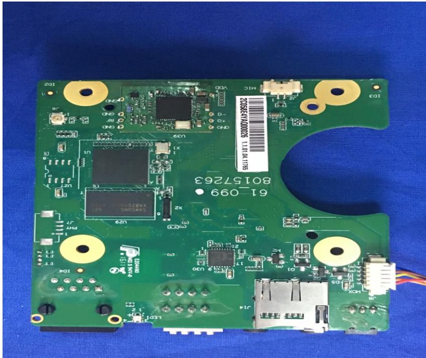
(5) EUT Photo
