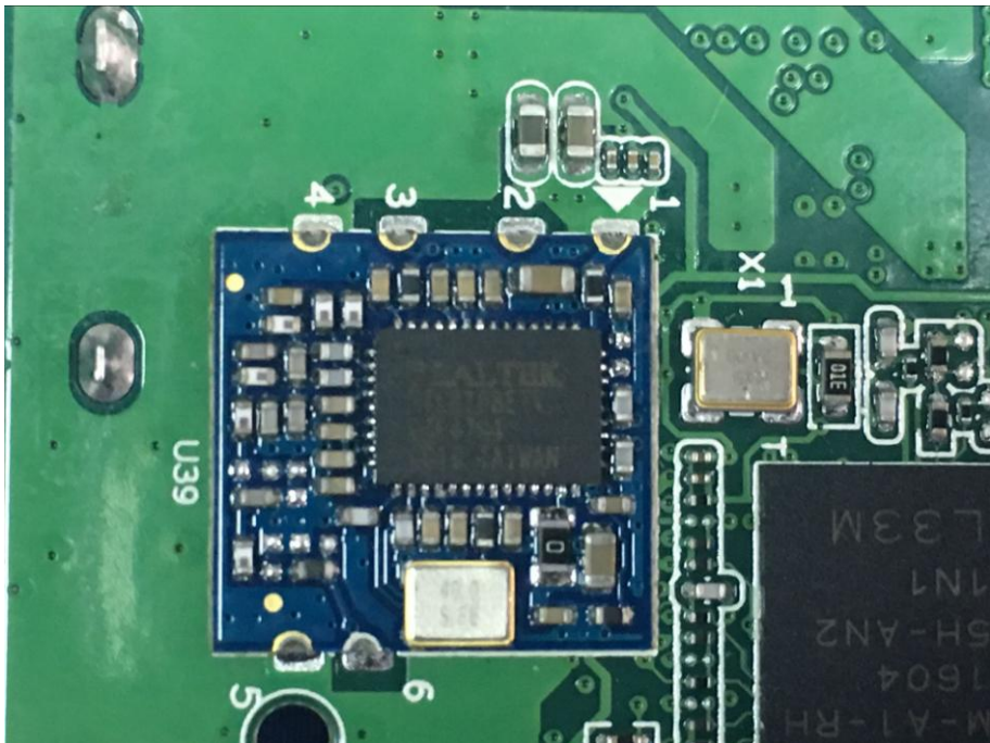
(4) EUT Photo
