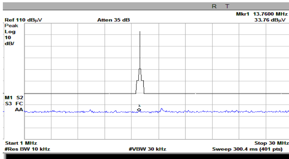
(Plot A: Test Antenna Vertical)
