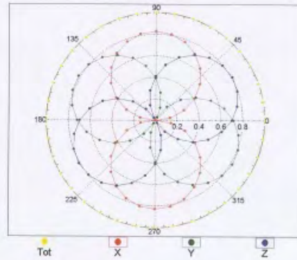
f=1800 MHz,R22
