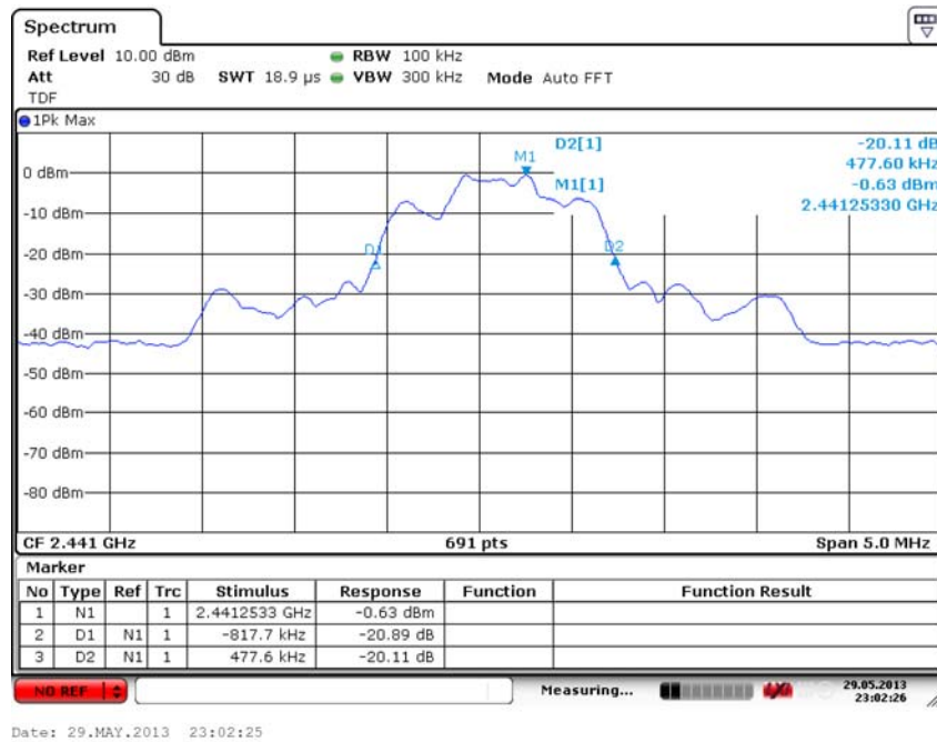
Fig. 52 Occupied 20dB Bandwidth ( \pi/4 DQPSK, Ch 39)
