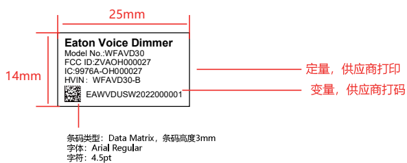
粘贴示意图
