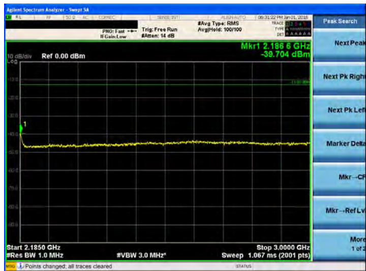
1GHz ~ 3GHz-4
