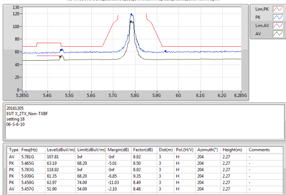
RE TX above 1GHz;Band:5.8G;11a;BWch:20MHz;Nss:1;Nant:2;Ch:5785MHz;TX
