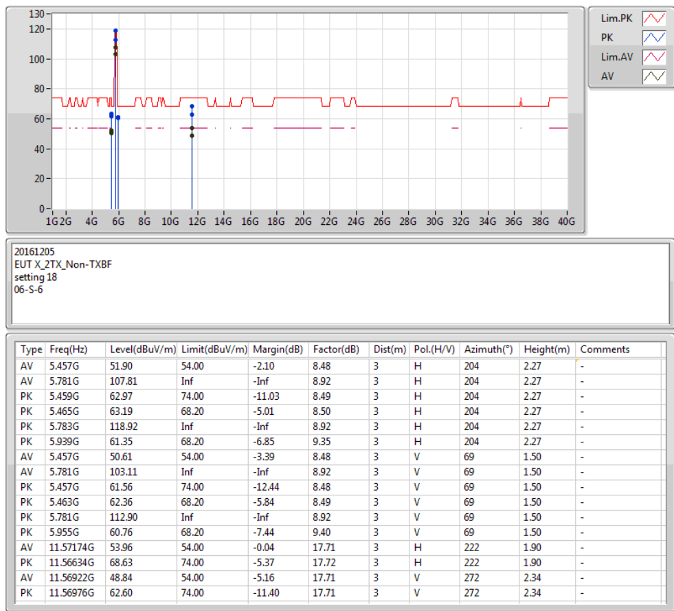
RE TX above 1GHz;Band:5.8G;11a;BWch:20MHz;Nss:1;Nant:2;Ch:5785MHz;TX
