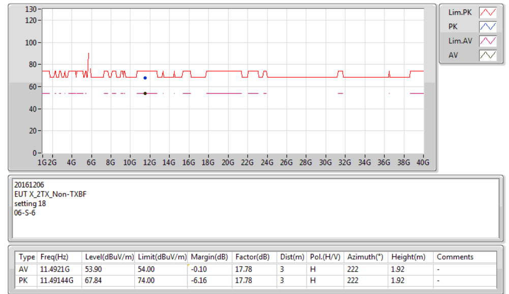
RE TX above 1GHz;Band:5.8G;11a;BWch:20MHz;Nss:1;Nant:2;Ch:5745MHz;TX
