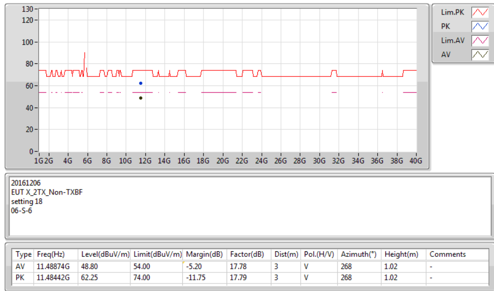
RE TX above 1GHz;Band:5.8G;11a;BWch:20MHz;Nss:1;Nant:2;Ch:5745MHz;TX
