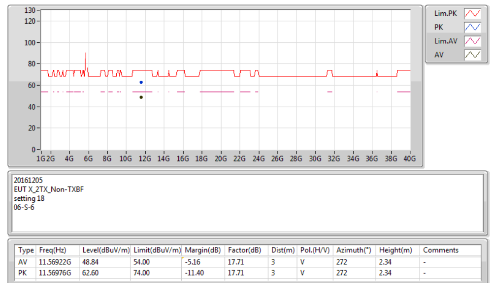
RE TX above 1GHz;Band:5.8G;11a;BWch:20MHz;Nss:1;Nant:2;Ch:5785MHz;TX
