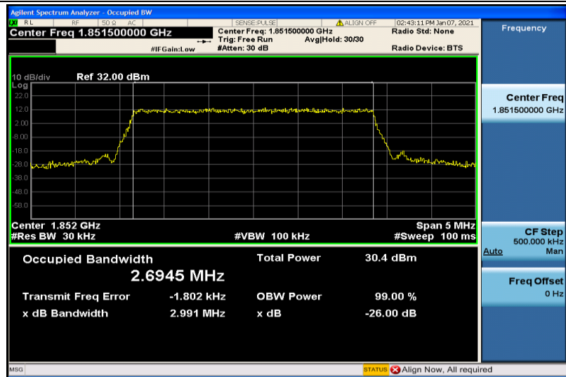
Band2-3MHz-QPSK-18615-15RB#0-2.6945
