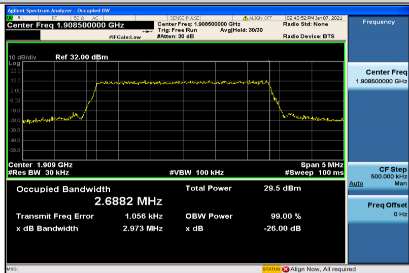
Band2-3MHz-QPSK-19185-15RB#0-2.6882
