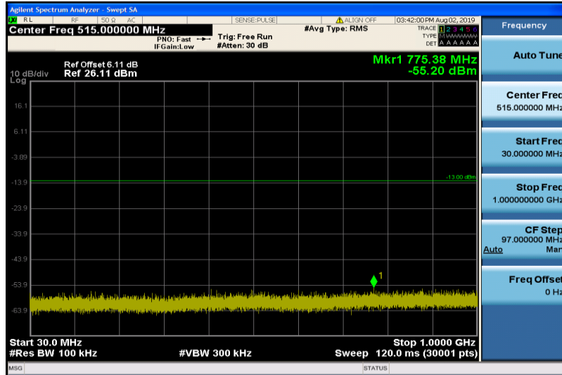
Band4-20MHz-QPSK-20050-1RB#0-30~1000MHz
