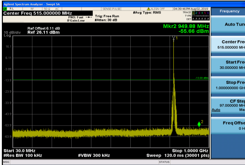
Band5-5MHz-QPSK-20425-1RB#0-30~1000MHz
