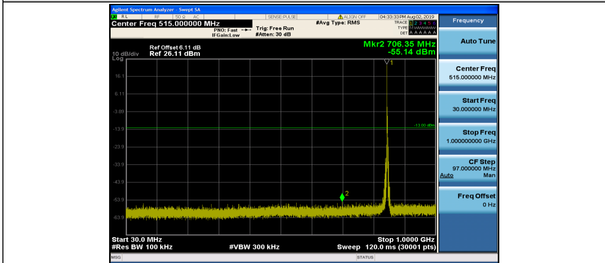
Band5-3MHz-QPSK-20635-1RB#0-30~1000MHz
