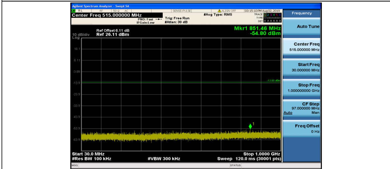
Band4-3MHz-QPSK-20385-1RB#0-30~1000MHz
