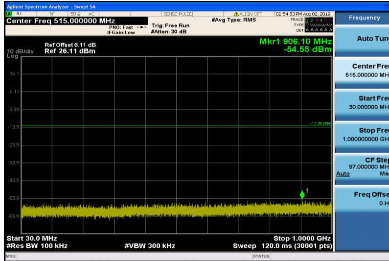
Band2-20MHz-16QAM-18700-1RB#0-30~1000MHz
