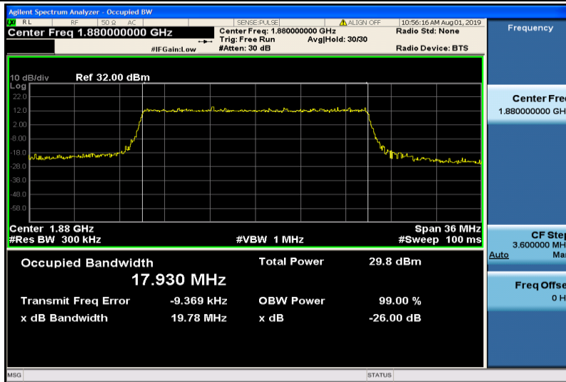
Band2-20MHz-QPSK-18900-100RB#0-17.930
