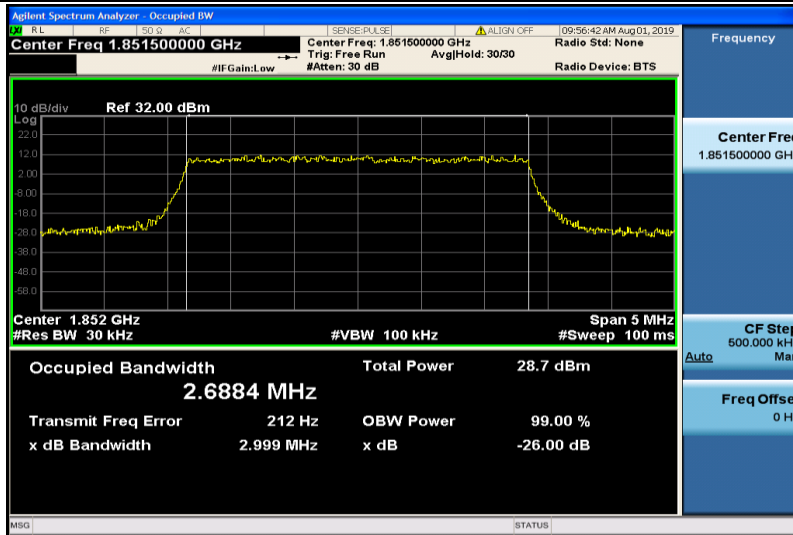
Band2-3MHz-QPSK-18615-15RB#0-2.6884
