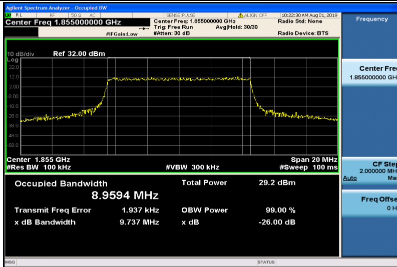
Band2-10MHz-QPSK-18550-50RB#0-8.9594
