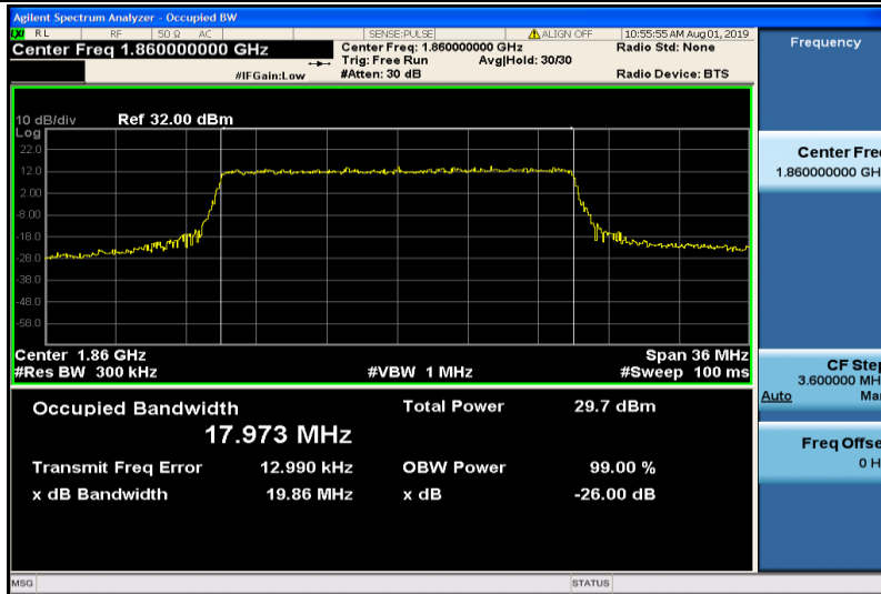
Band2-20MHz-QPSK-18700-100RB#0-17.973
