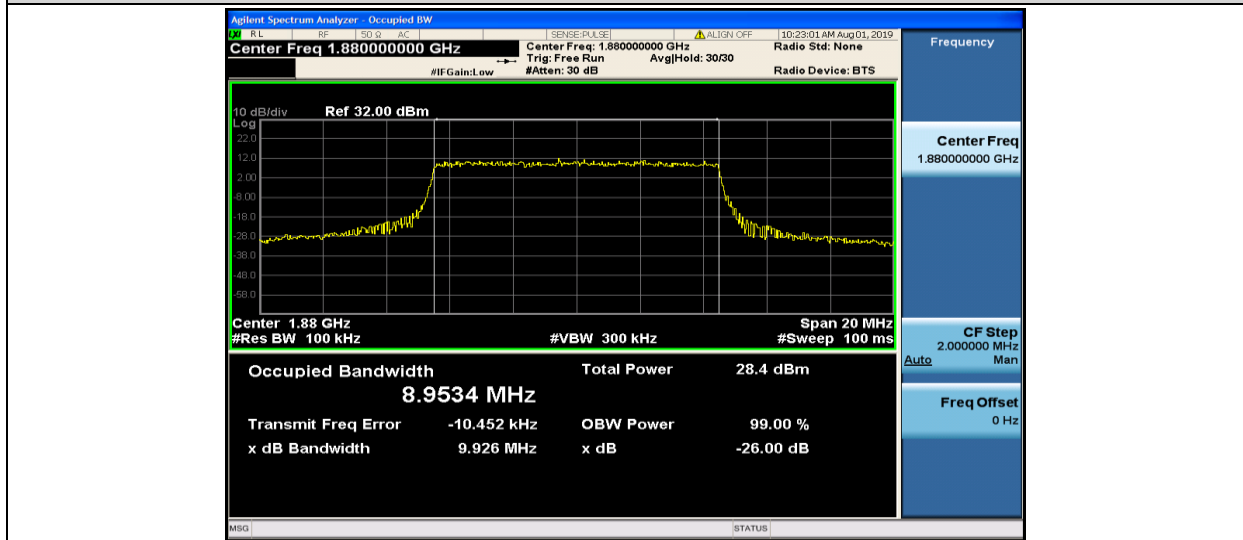
Band2-10MHz-16QAM-18900-50RB#0-8.9534
