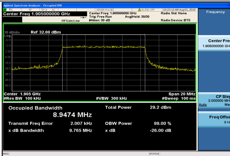
Band2-10MHz-QPSK-19150-50RB#0-8.9474
