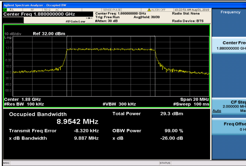
Band2-10MHz-QPSK-18900-50RB#0-8.9542
