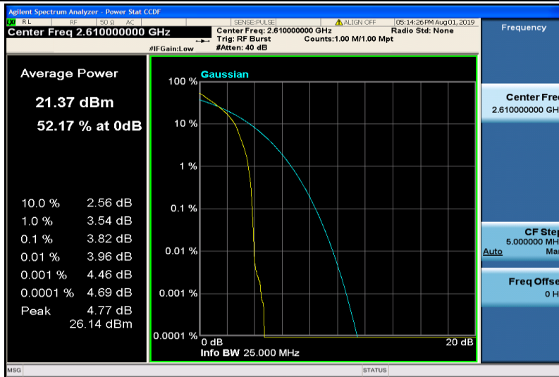
Band38-20MHz-QPSK-38150-1RB#0
