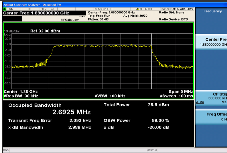
Band2-3MHz-QPSK-18900-15RB#0-2.6925
