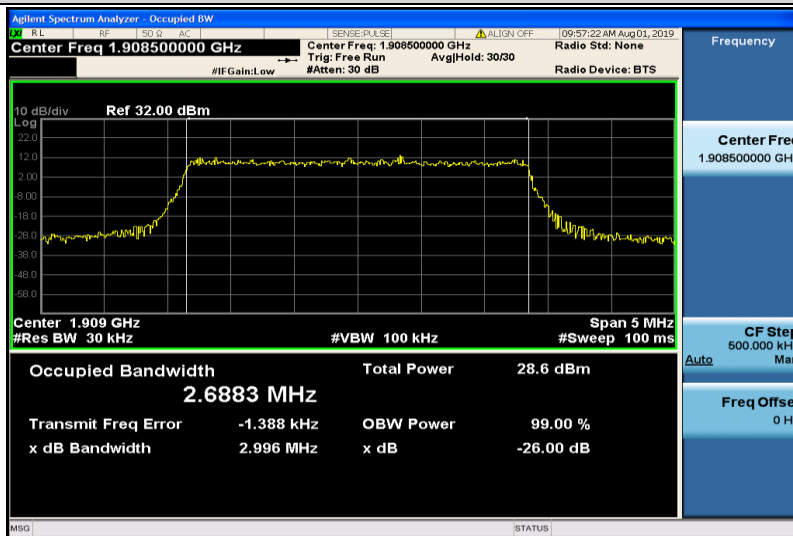
Band2-3MHz-QPSK-19185-15RB#0-2.6883
