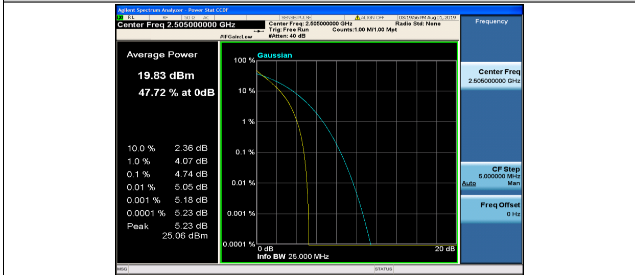
Band7-10MHz-QPSK-20800-50RB#0
