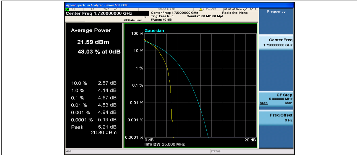
Band4-20MHz-QPSK-20050-1RB#0
