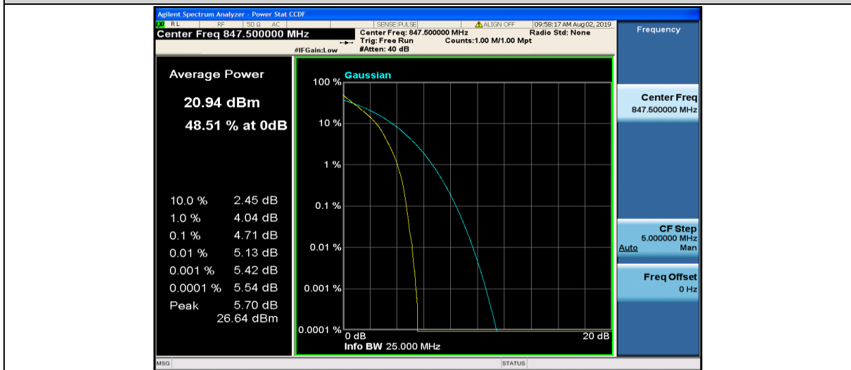
Band5-3MHz-QPSK-20635-15RB#0
