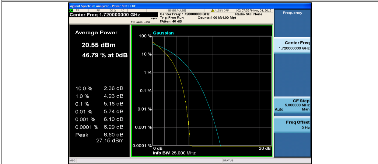
Band4-20MHz-QPSK-20050-100RB#0
