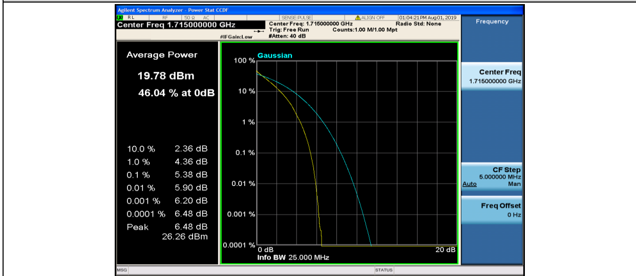
Band4-10MHz-QPSK-20000-50RB#0
