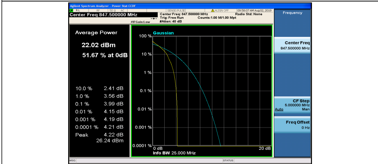
Band5-3MHz-QPSK-20635-1RB#0
