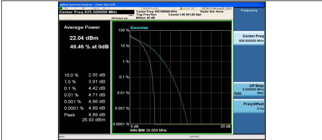
Band5-3MHz-QPSK-20415-1RB#0
