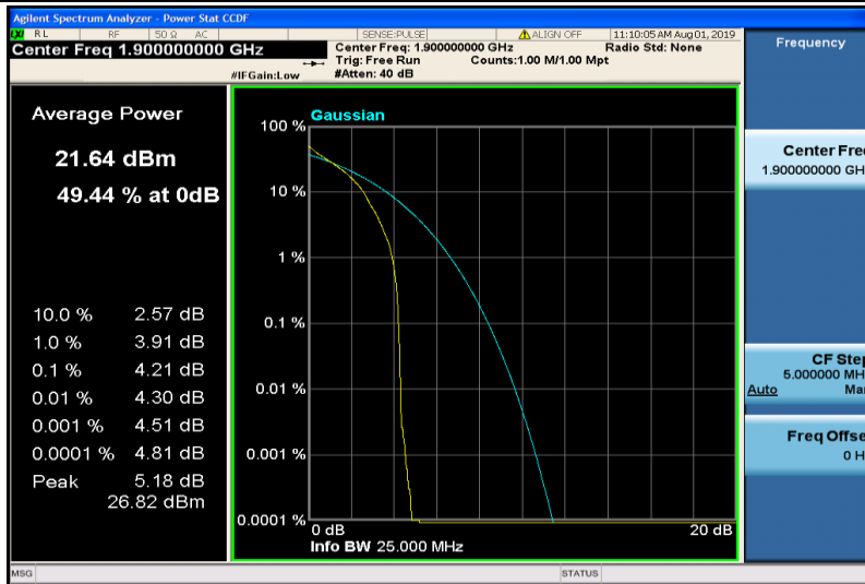
Band2-20MHz-QPSK-19100-1RB#0
