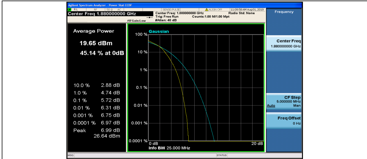
Band2-20MHz-16QAM-18900-100RB#0
