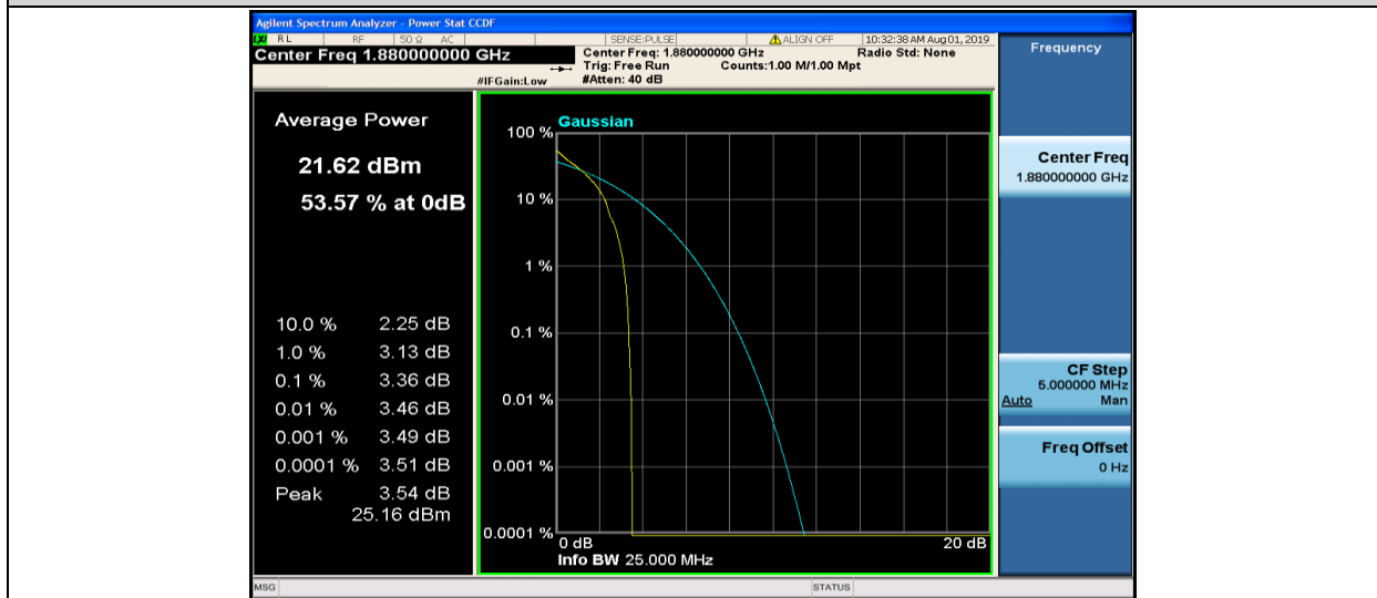
Band2-10MHz-QPSK-18900-1RB#0
