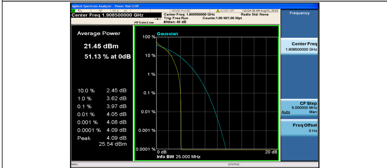
Band2-3MHz-QPSK-19185-1RB#0
