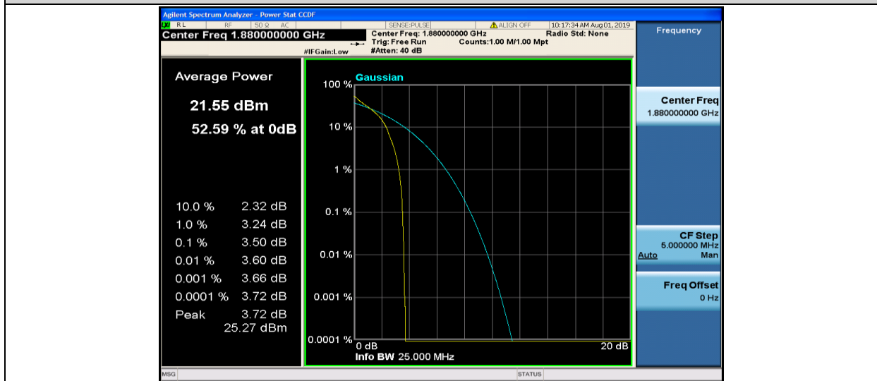
Band2-5MHz-QPSK-18900-1RB#0
