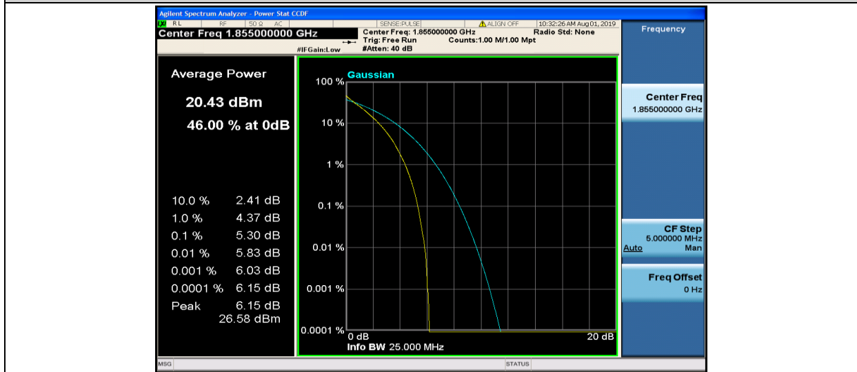
Band2-10MHz-QPSK-18650-50RB#0
