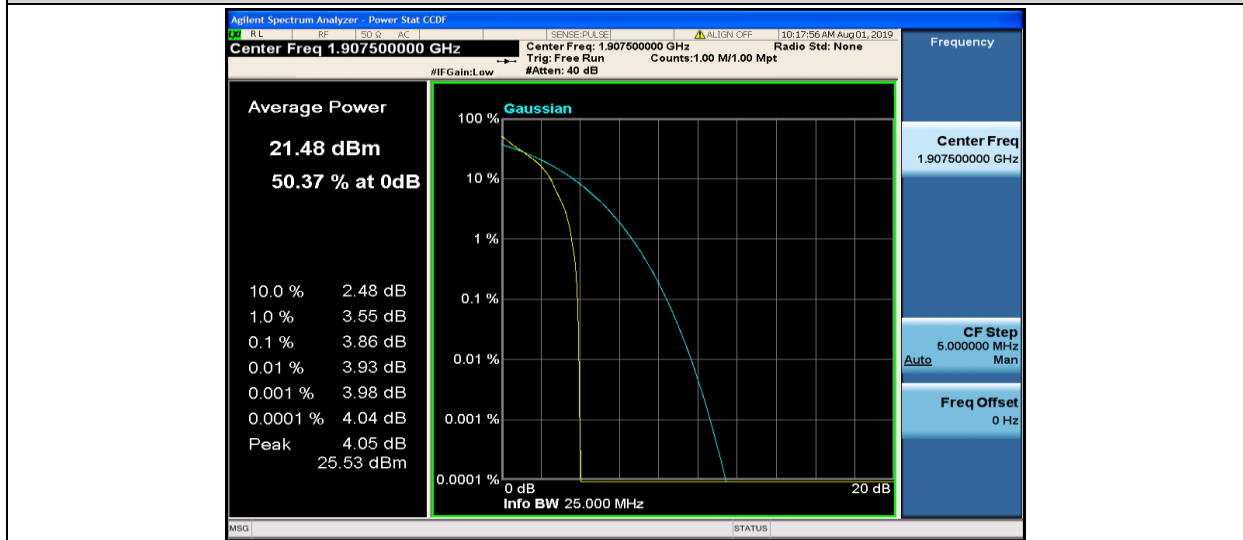
Band2-5MHz-QPSK-19175-1RB#0
