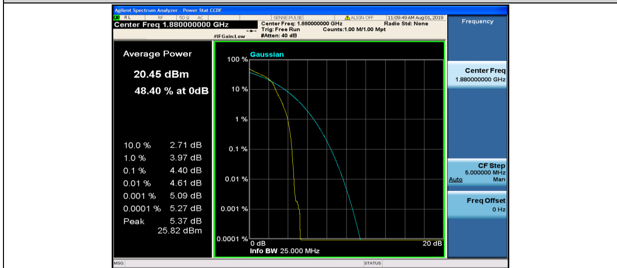
Band2-20MHz-16QAM-18900-1RB#0
