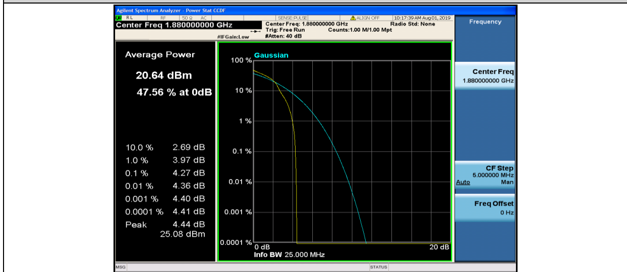
Band2-5MHz-16QAM-18900-1RB#0
