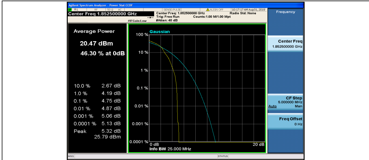
Band2-5MHz-16QAM-18625-1RB#0
