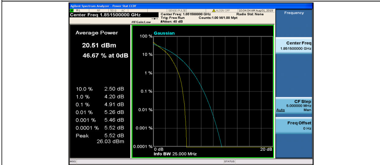
Band2-3MHz-QPSK-18615-15RB#0
