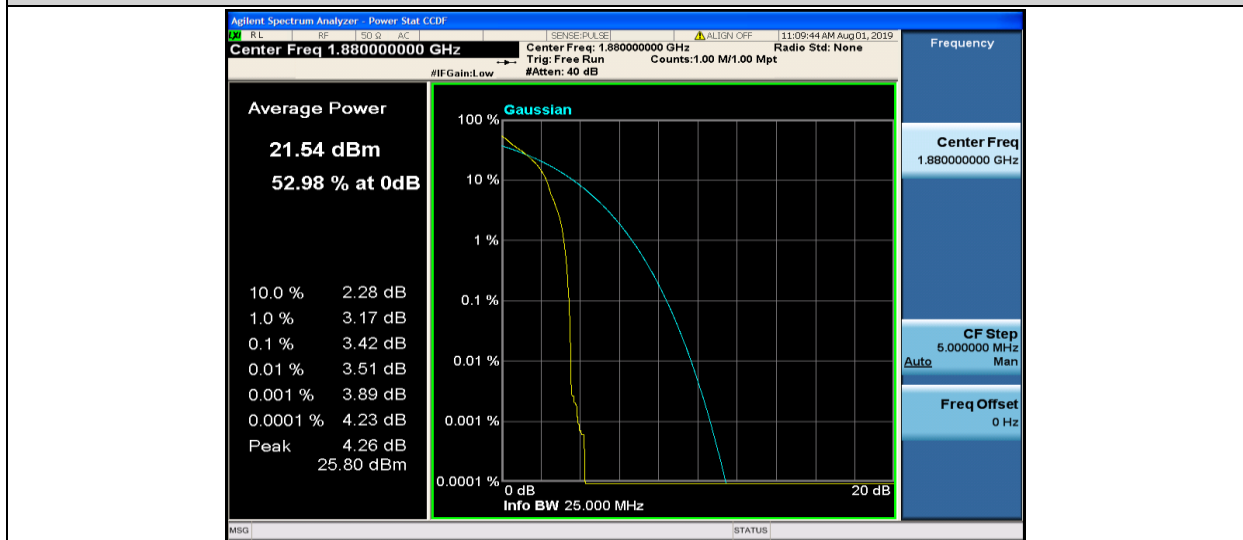
Band2-20MHz-QPSK-18900-1RB#0
