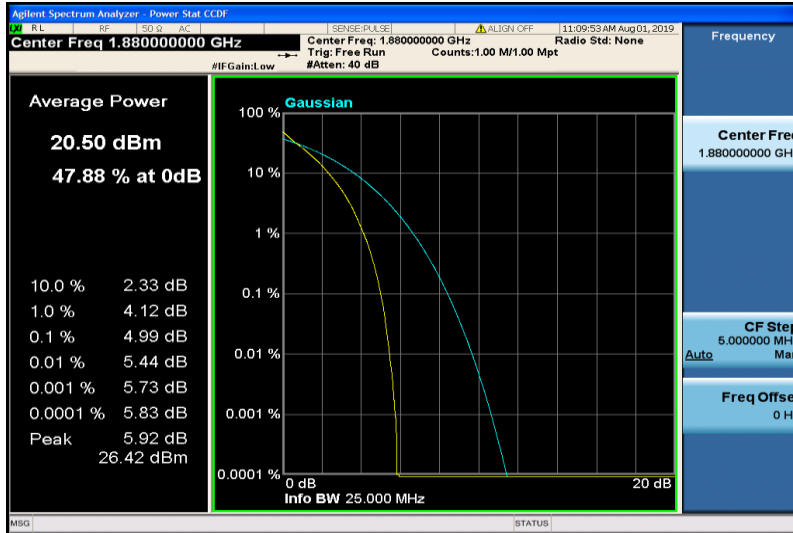
Band2-20MHz-QPSK-18900-100RB#0
