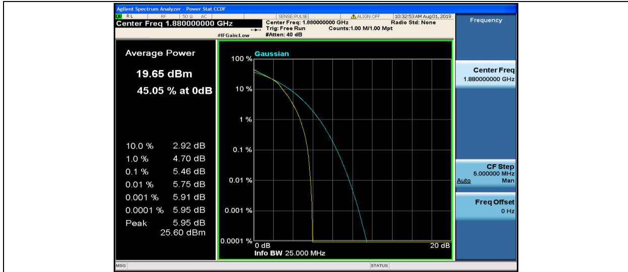
Band2-10MHz-16QAM-18900-50RB#0
