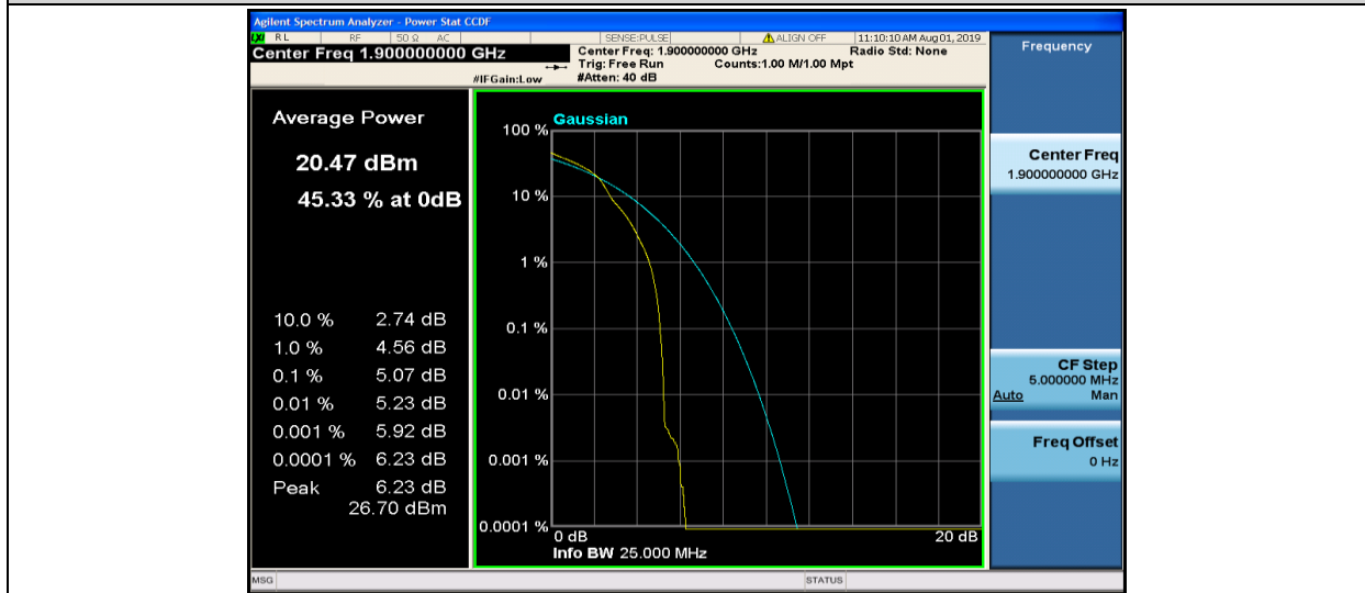
Band2-20MHz-16QAM-19100-1RB#0
