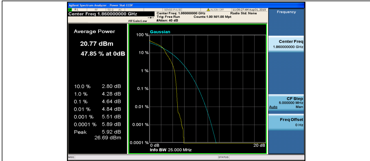
Band2-20MHz-16QAM-18700-1RB#0
