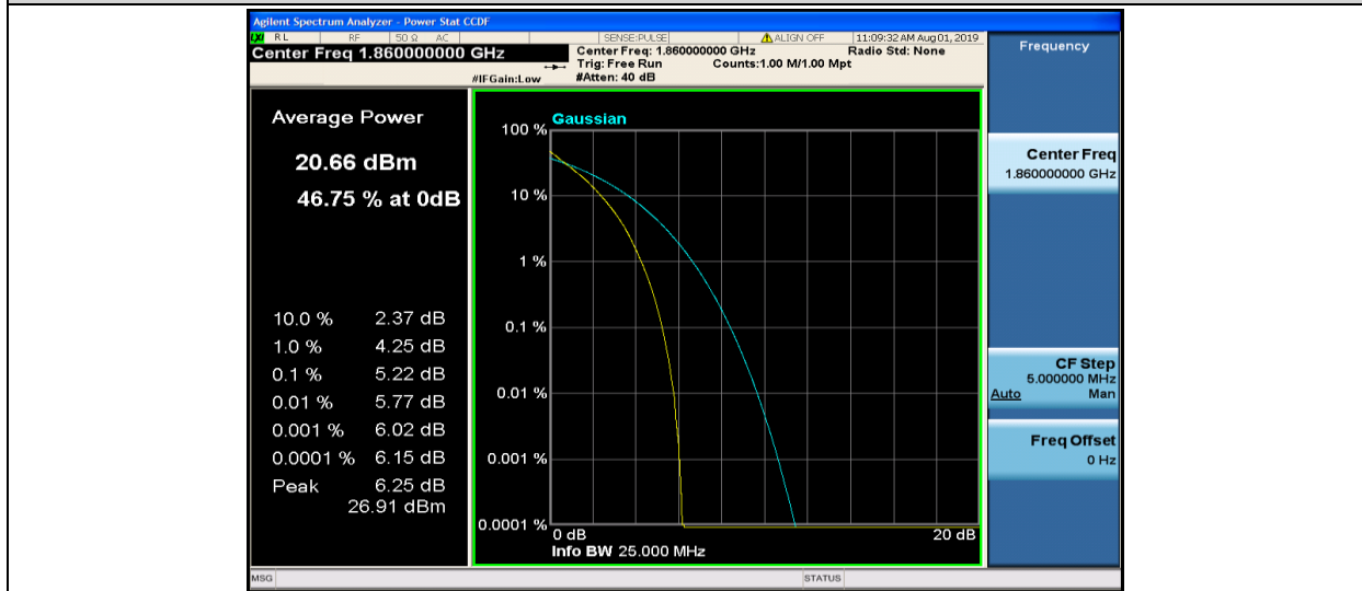
Band2-20MHz-QPSK-18700-100RB#0
