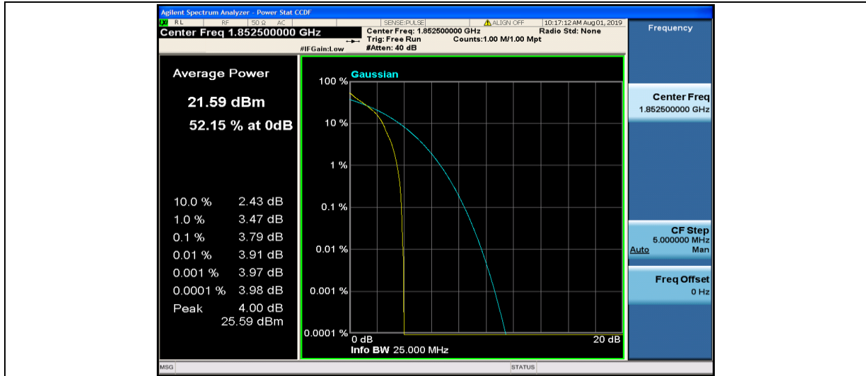
Band2-5MHz-QPSK-18625-1RB#0
