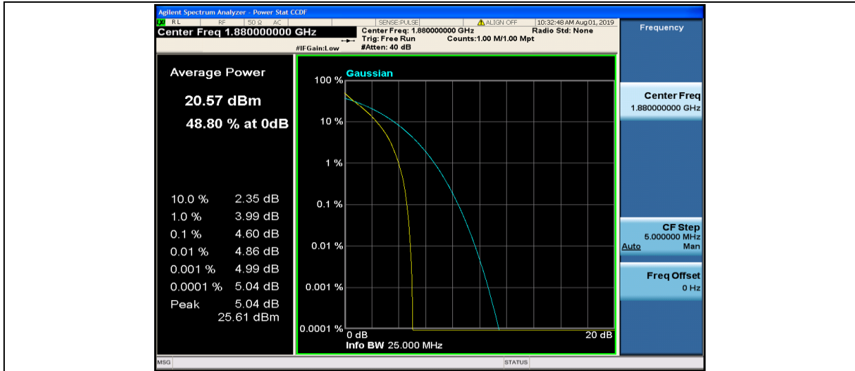
Band2-10MHz-QPSK-18900-50RB#0
