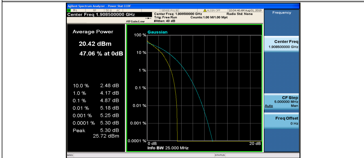
Band2-3MHz-QPSK-19185-15RB#0
