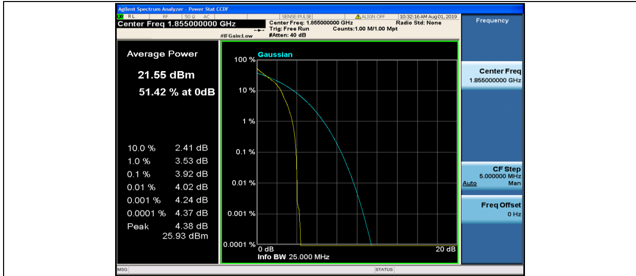
Band2-10MHz-QPSK-18650-1RB#0
