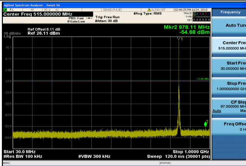
Band5-3MHz-QPSK-20635-1RB#0-30~1000MHz
