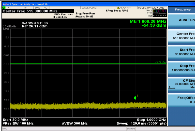
Band2-20MHz-QPSK-19100-1RB#0-30~1000MHz
