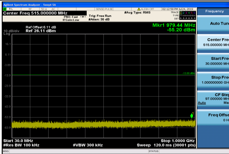
Band4-5MHz-QPSK-20375-1RB#0-30~1000MHz
