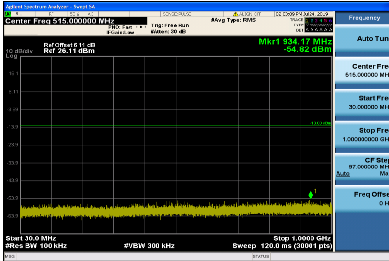
Band4-3MHz-QPSK-19965-1RB#0-30~1000MHz
