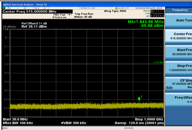
Band2-20MHz-QPSK-18900-1RB#0-30~1000MHz
