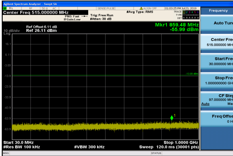
Band2-20MHz-16QAM-18700-1RB#0-30~1000MHz
