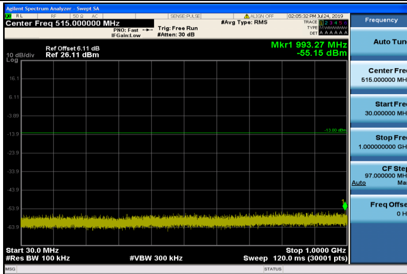
Band4-3MHz-QPSK-20385-1RB#0-30~1000MHz
