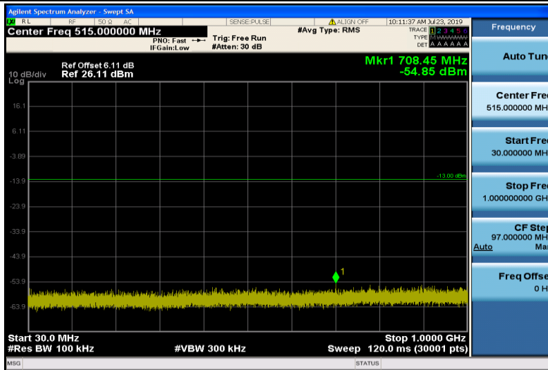
Band2-10MHz-QPSK-19150-1RB#0-30~1000MHz
