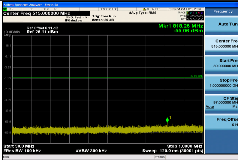
Band2-20MHz-QPSK-18700-1RB#0-30~1000MHz
