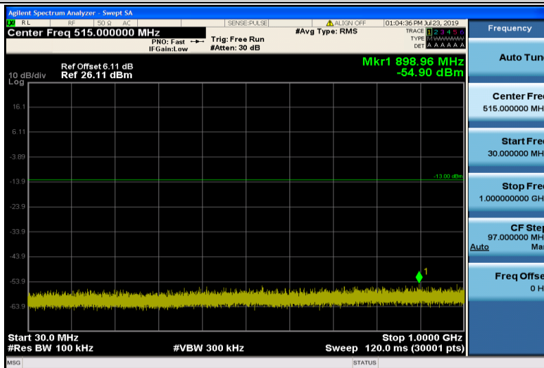
Band2-20MHz-16QAM-18900-1RB#0-30~1000MHz
