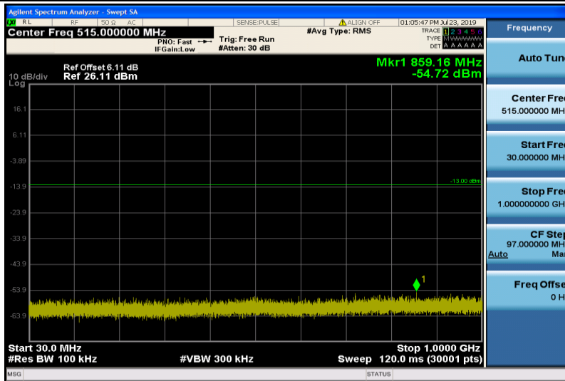
Band2-20MHz-16QAM-19100-1RB#0-30~1000MHz
