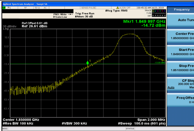
Band2-5MHz-QPSK-18625-1RB#0
