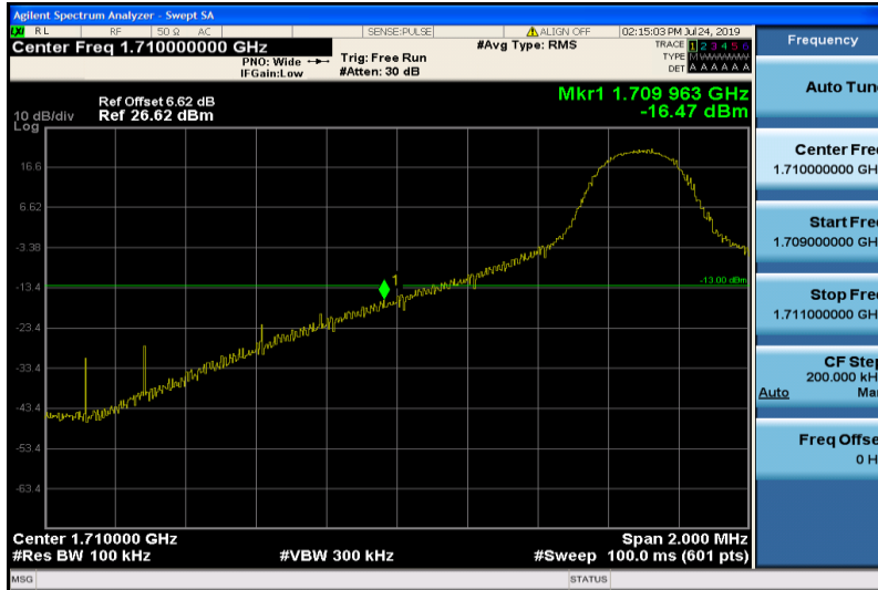
Band4-10MHz-QPSK-20000-1RB#0
