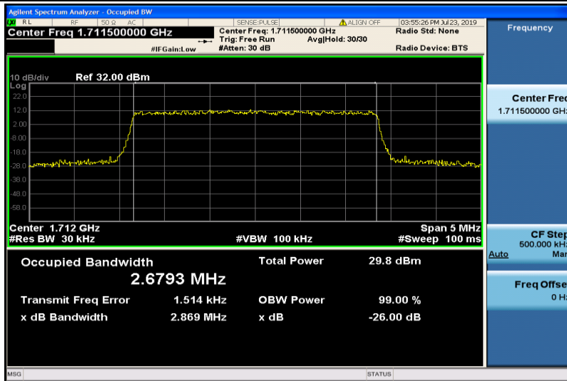
Band4-3MHz-QPSK-19965-15RB#0-2.6793
