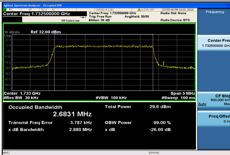
Band4-3MHz-QPSK-20175-15RB#0-2.6831
