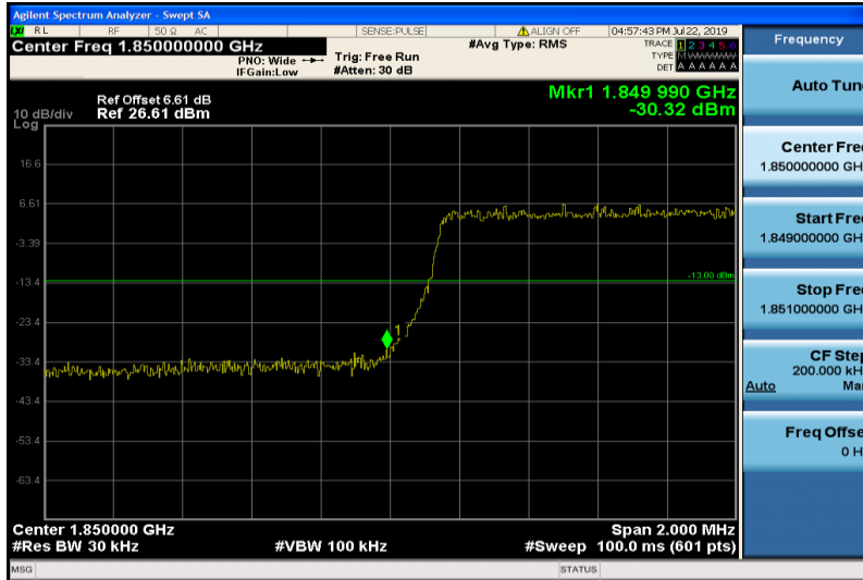
Band2-3MHz-QPSK-18615-15RB#0
