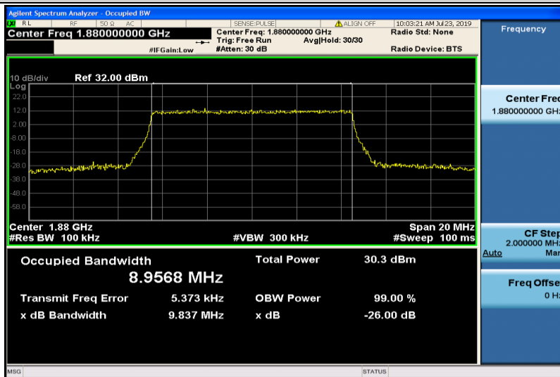
Band2-10MHz-QPSK-18900-50RB#0-8.9568
