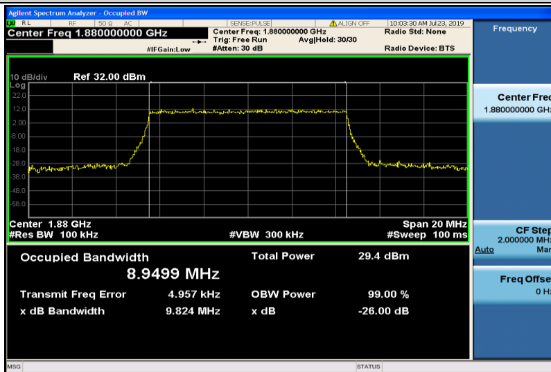
Band2-10MHz-16QAM-18900-50RB#0-8.9499
