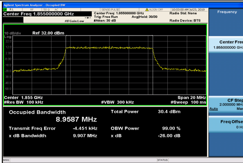
Band2-10MHz-QPSK-18650-50RB#0-8.9587
