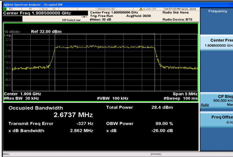
Band2-3MHz-QPSK-19185-15RB#0-2.6737
