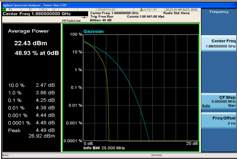
Band2-10MHz-QPSK-18900-1RB#0
