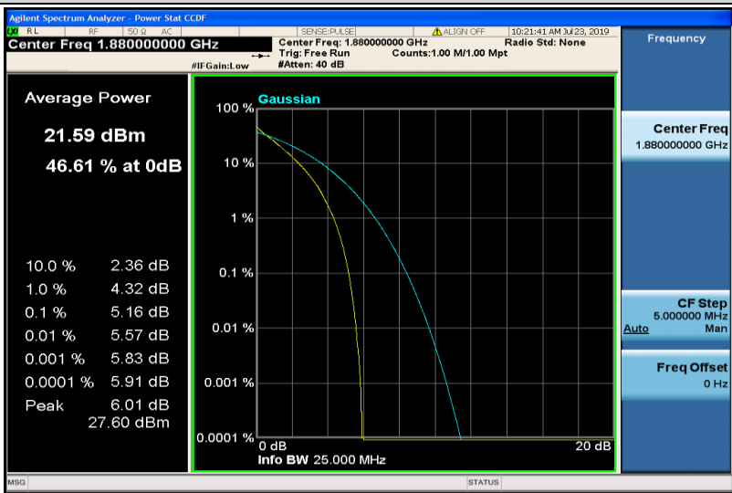
Band2-10MHz-QPSK-18900-50RB#0
