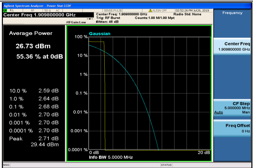
GPRS1900-810
