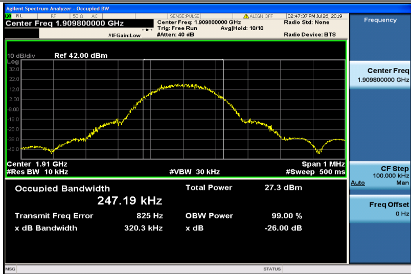
GPRS1900-810
