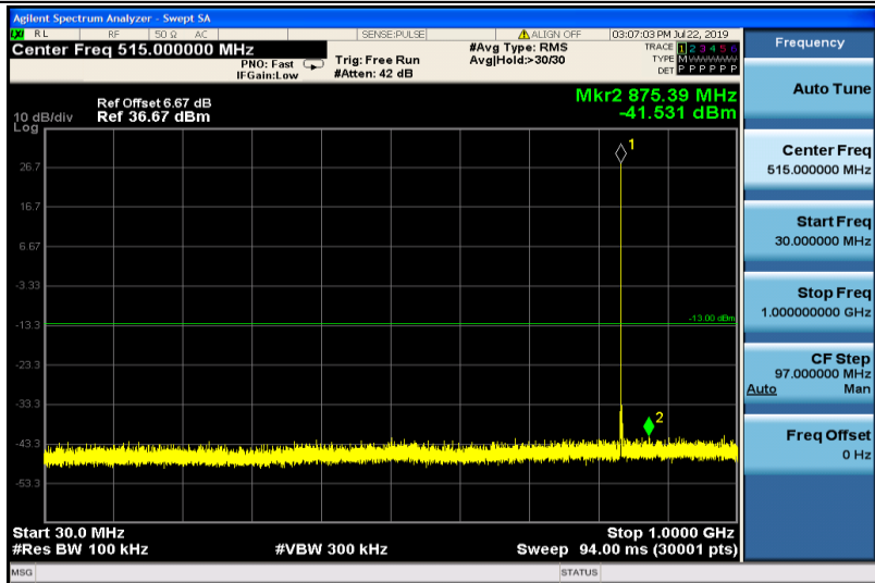
EGPRS850-190-30~1000
