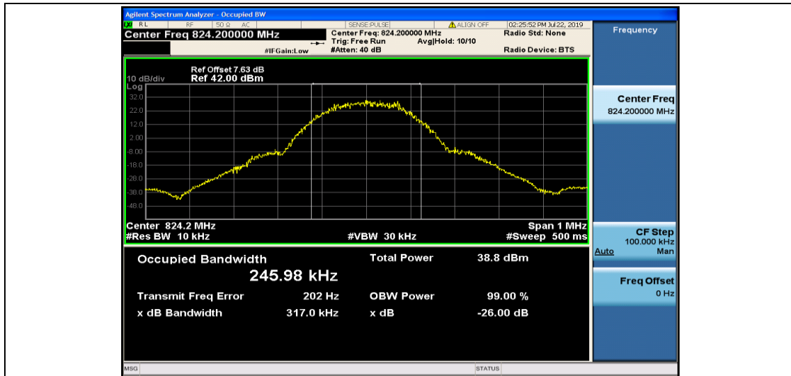
GSM850-128
