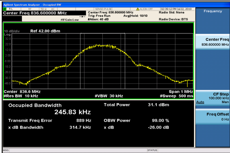
GPRS850-190
