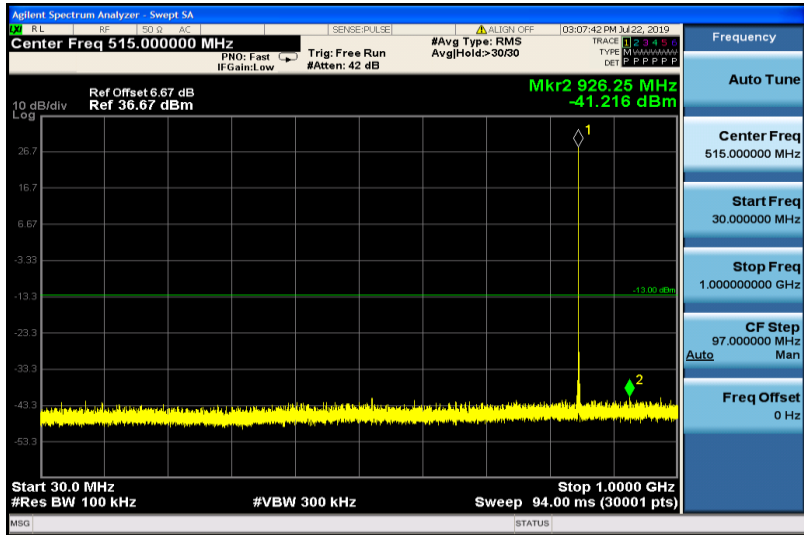
EGPRS850-251-30~1000
