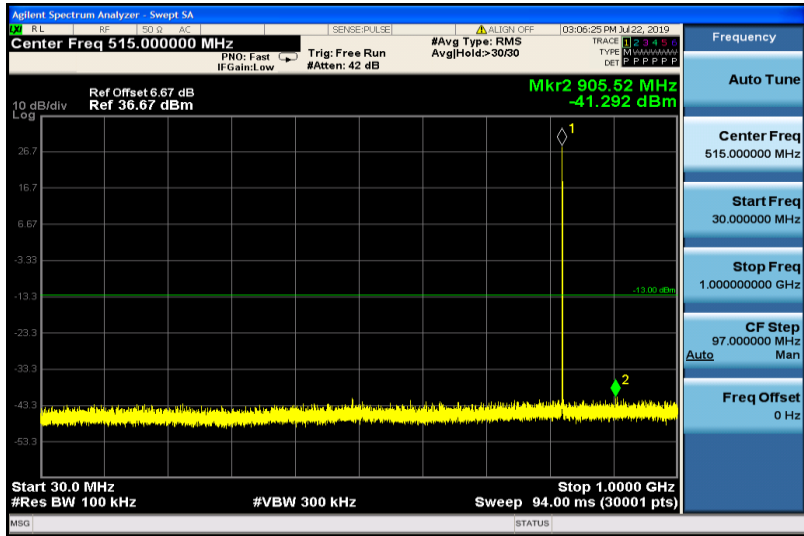
EGPRS850-128-30~1000
