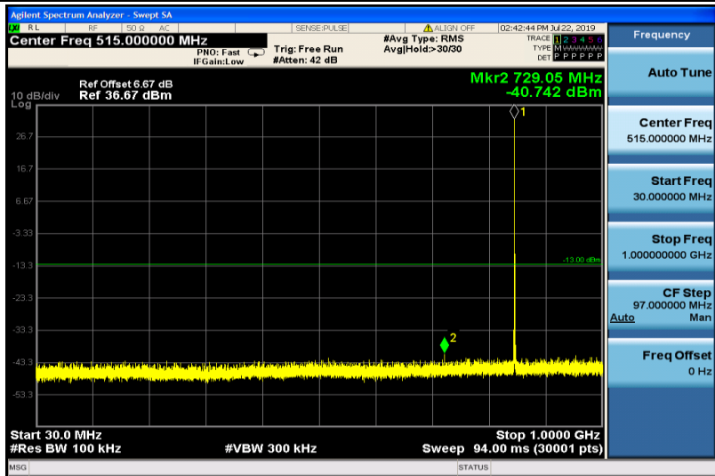
GPRS850-251-30~1000
