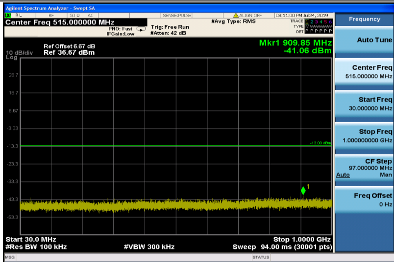
GSM1900-661-30~1000
