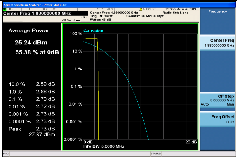
GSM1900-661
