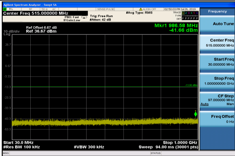
GPRS1900-661-30~1000
