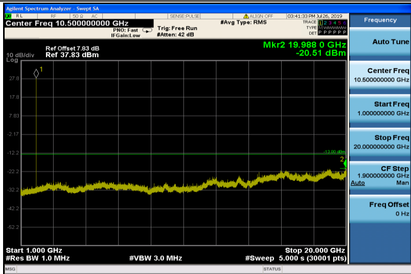
EGPRS1900-810-1000~20000
