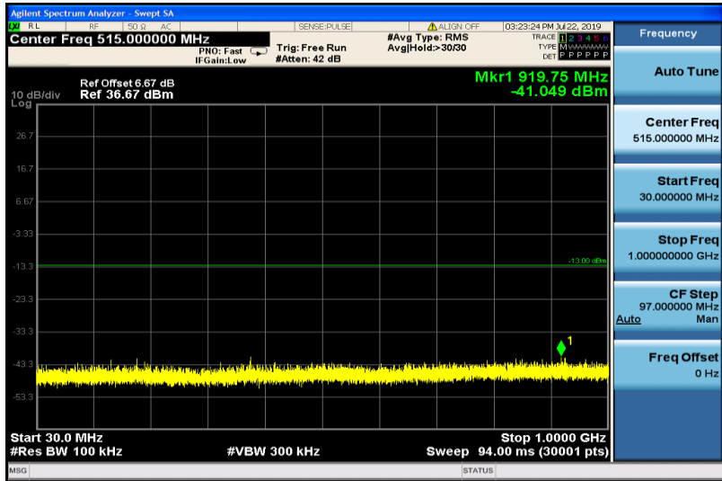
GSM1900-810-30~1000
