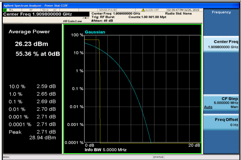
GSM1900-810
