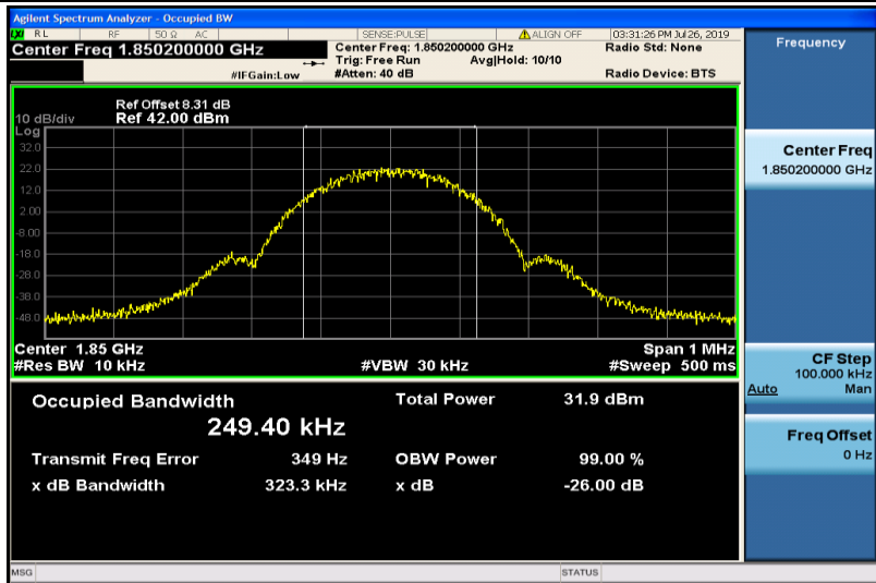
EGPRS1900-512
