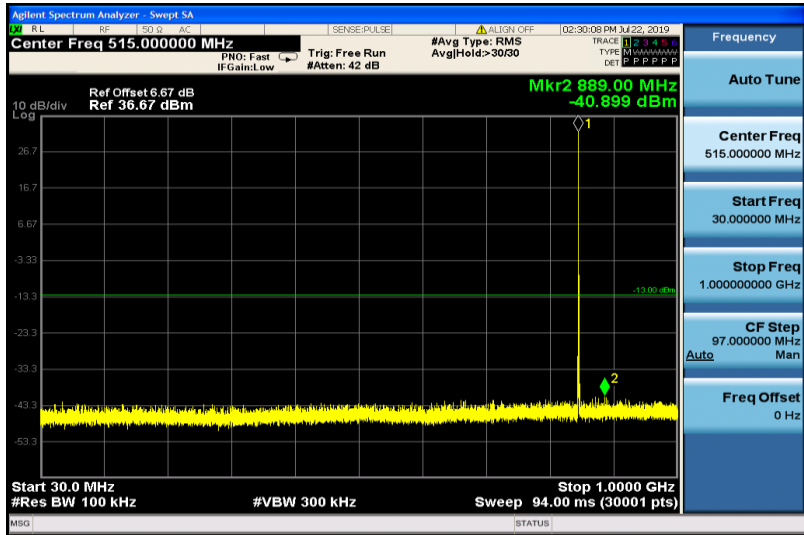
GSM850-251-30~1000
