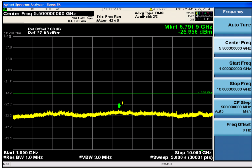
EGPRS850-190-1000~10000
