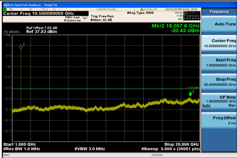
GPRS1900-810-1000~20000
