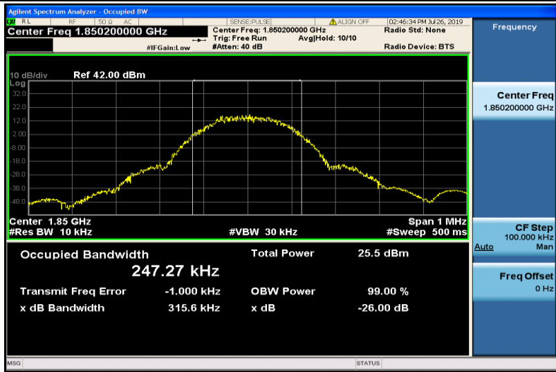
GPRS1900-512
