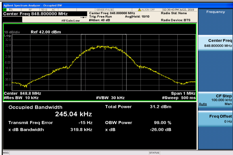
GPRS850-251
