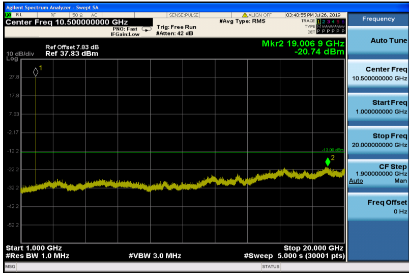
EGPRS1900-661-1000~20000
