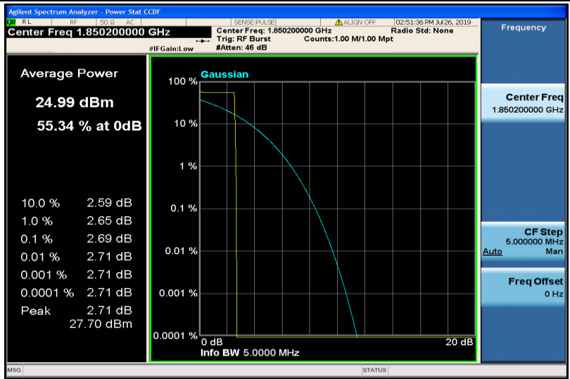
GPRS1900-512
