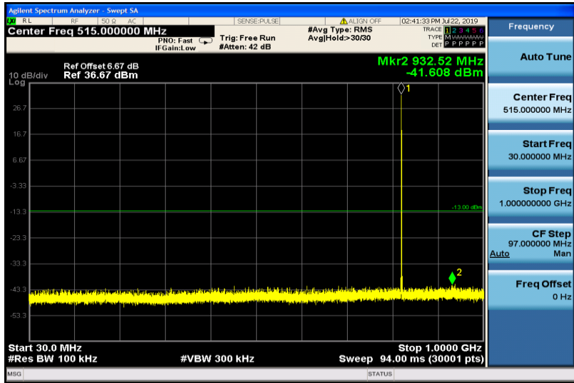
GPRS850-128-30~1000
