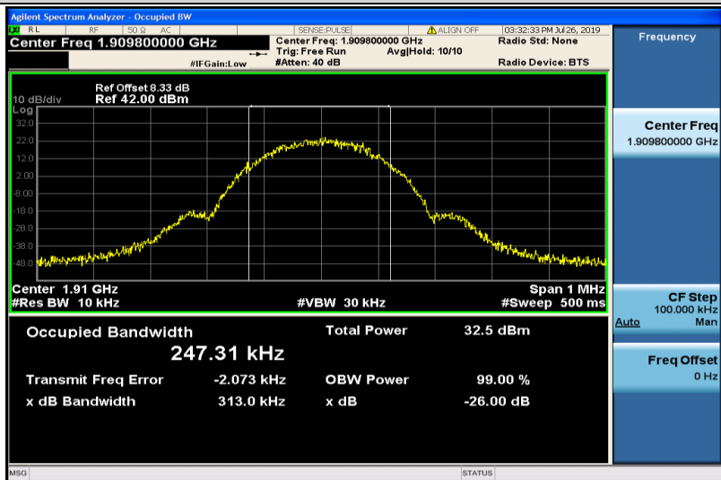
EGPRS1900-810
