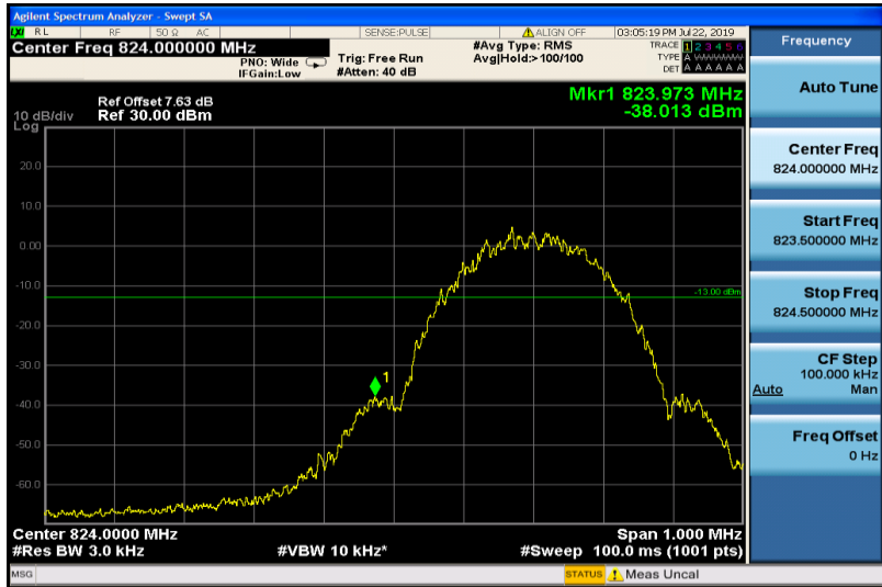
EGPRS850-128
