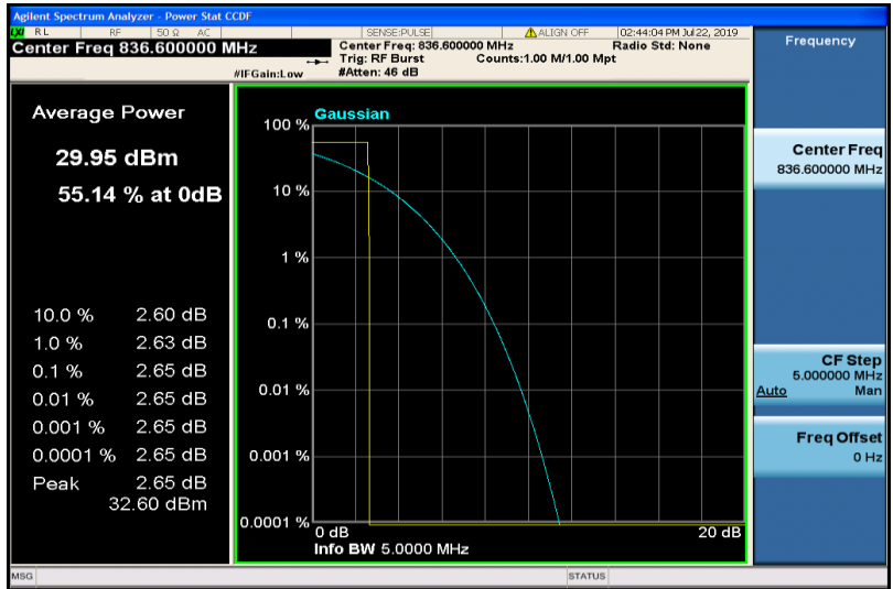
GPRS850-190
