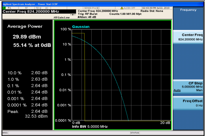
GPRS850-128
