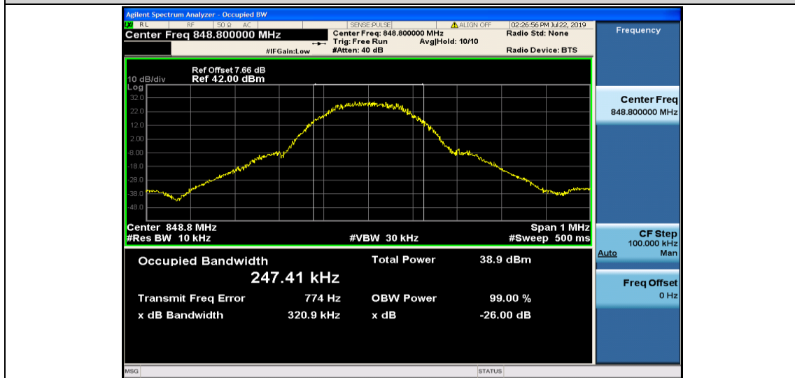
GSM850-251
