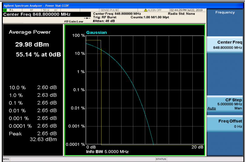
GPRS850-251
