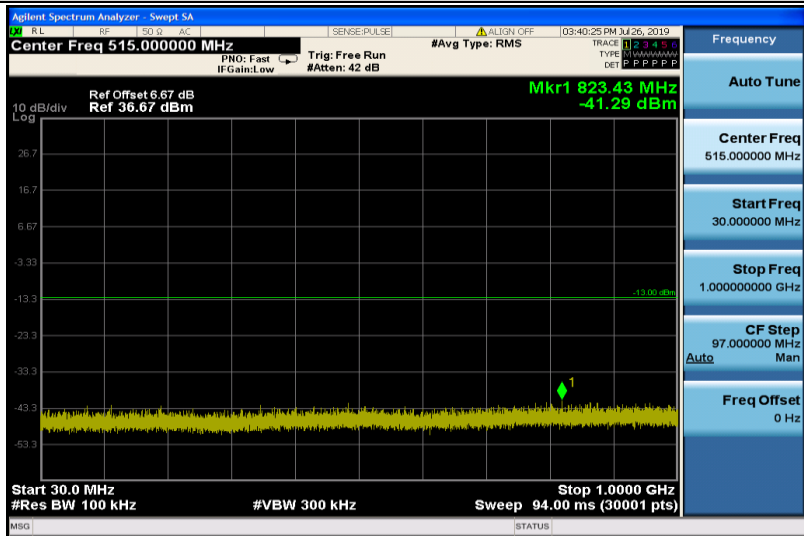
EGPRS1900-661-30~1000
