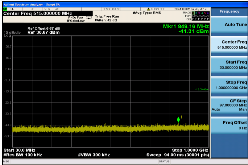
EGPRS1900-810-30~1000
