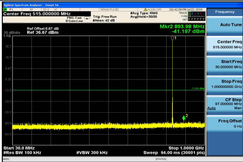
GPRS850-190-30~1000
