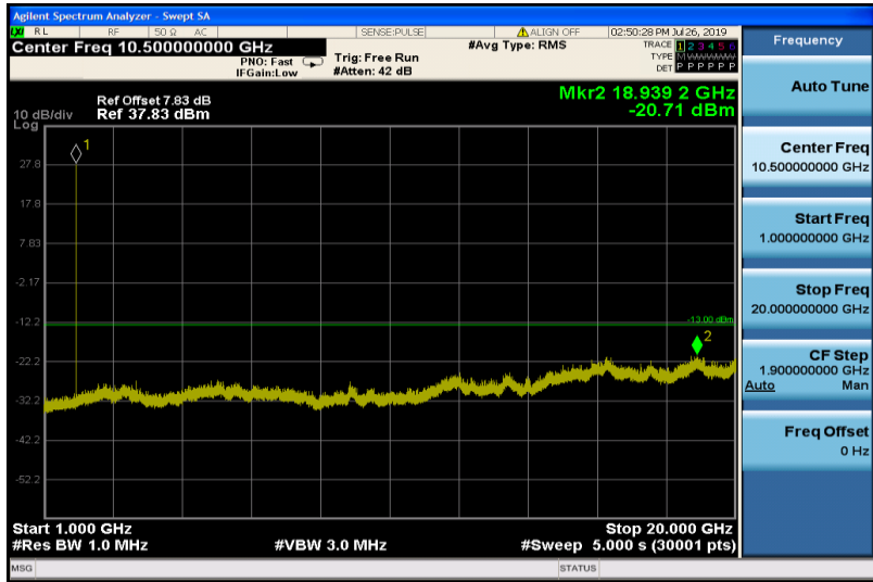
GPRS1900-661-1000~20000
