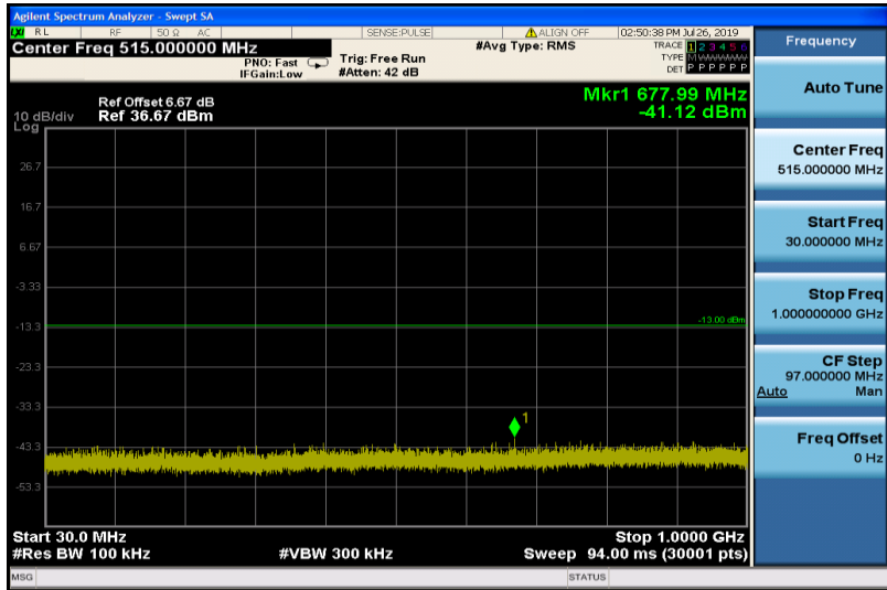
GPRS1900-810-30~1000
