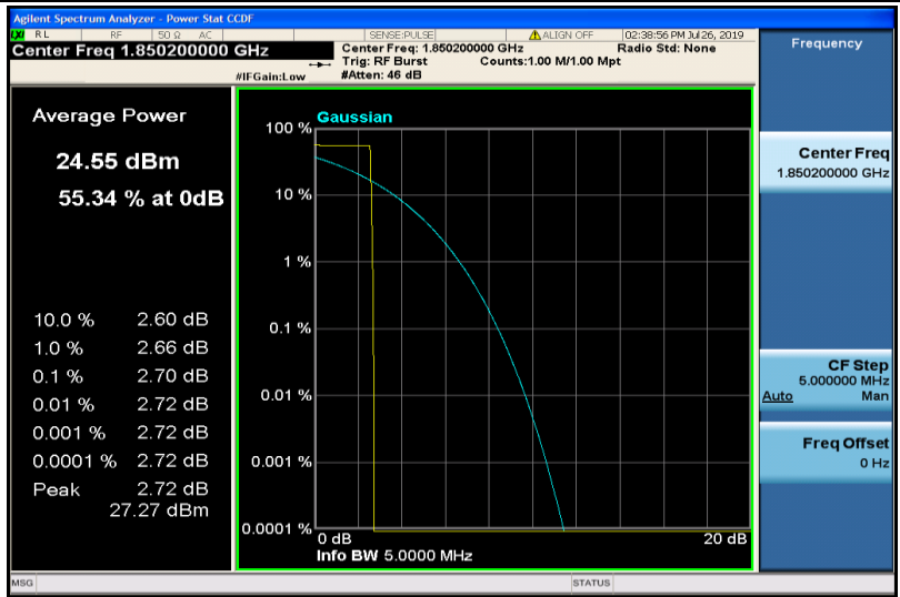
GSM1900-512
