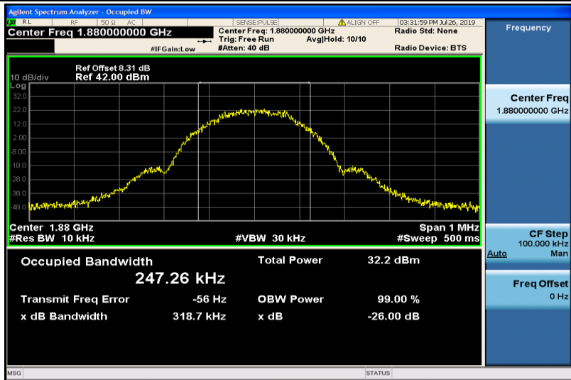
EGPRS1900-661
