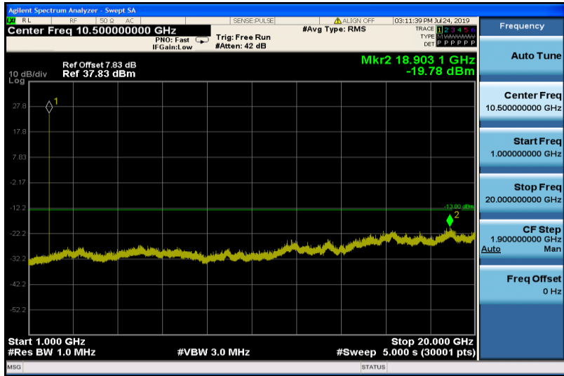
GSM1900-661-1000~20000
