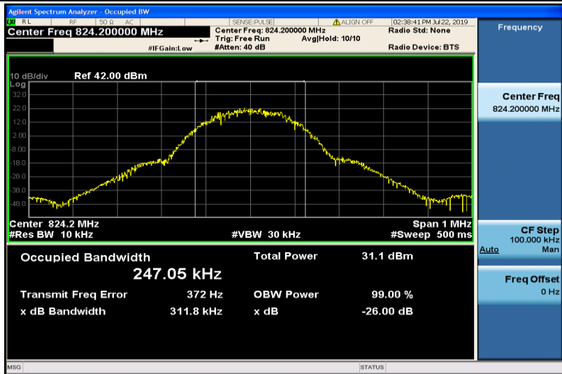
GPRS850-128
