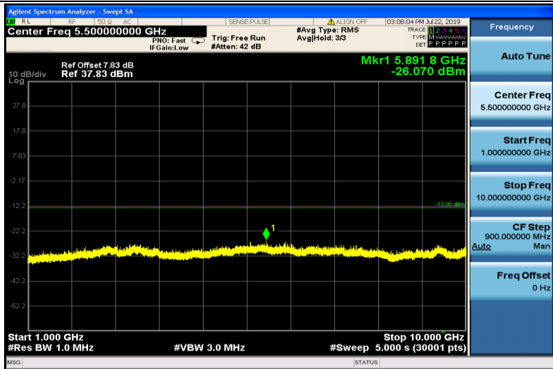
EGPRS850-251-1000~10000
