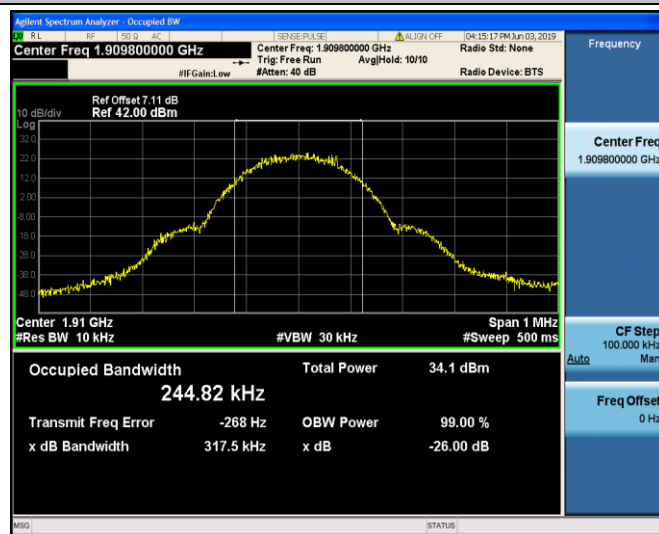
GPRS1900_810
