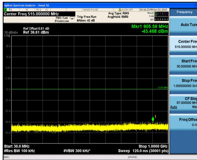
GPRS1900_810
