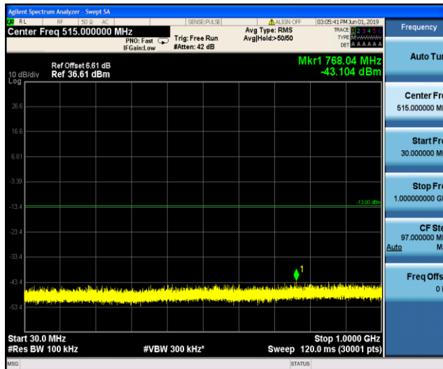
GSM1900_810
