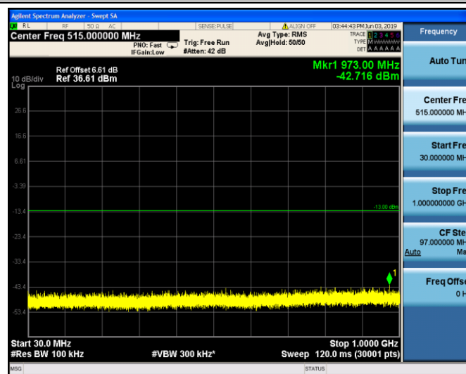
GPRS1900_661
