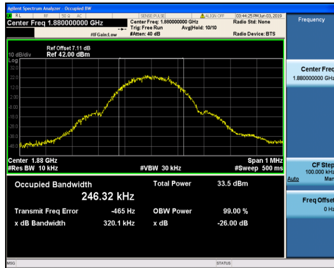
GPRS1900_661
