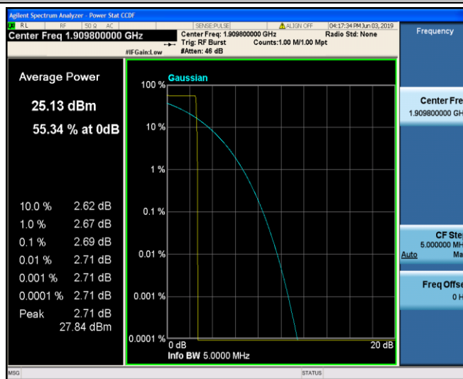
GPRS1900_810
