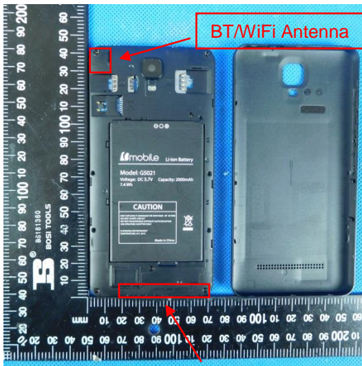
GSM/WCDMA/LTE Antenna
