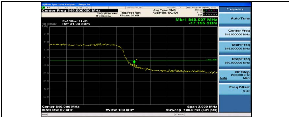
Band5_3MHz_16QAM_20635_15RB#0
