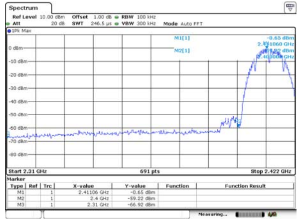
CH01-Bandedge
