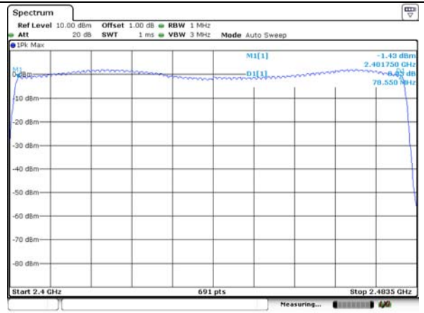
\pi/4 DQPSK
