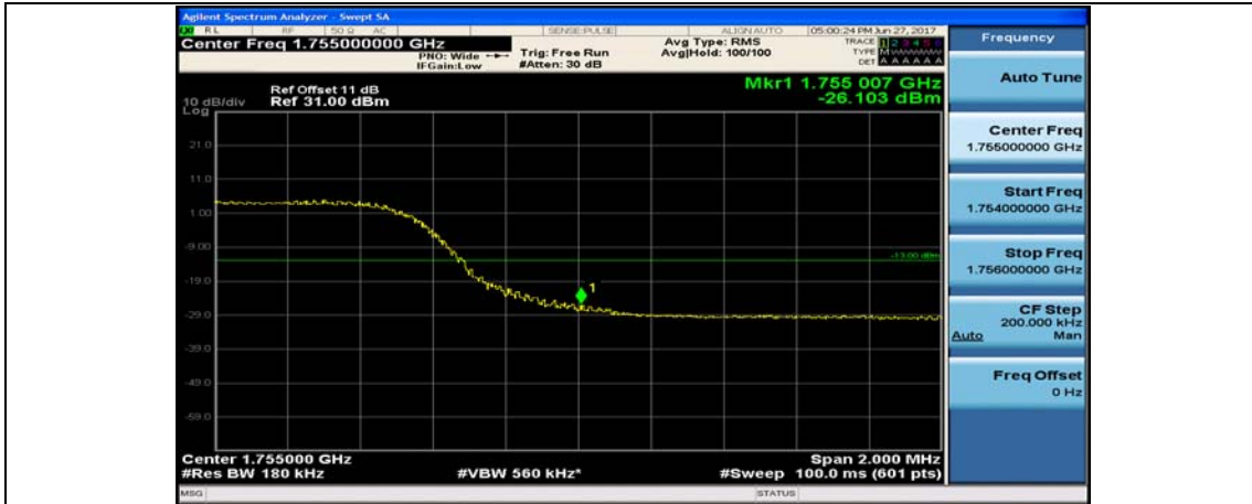
Band4_15MHz_QPSK_2025_75RB#0
