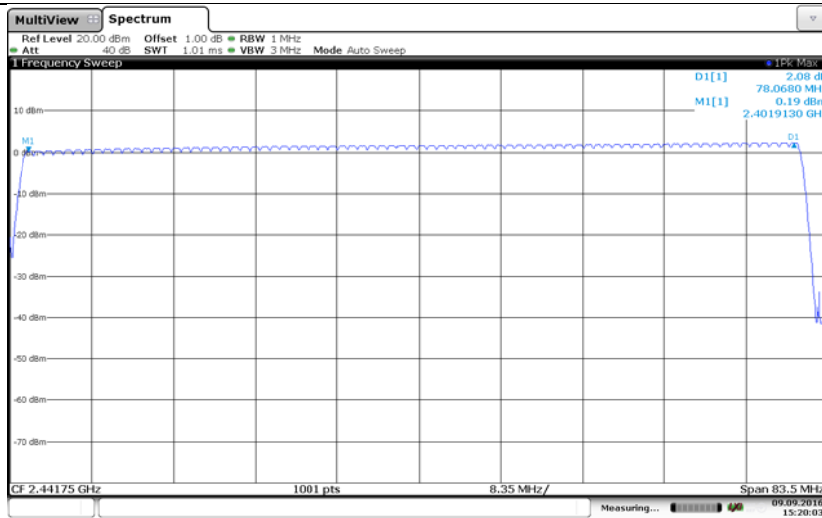
GFSK
