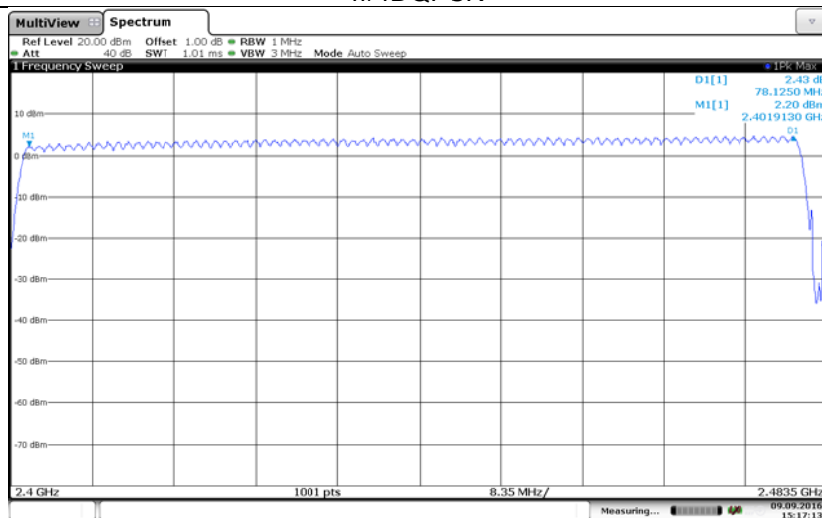
8DPSK
