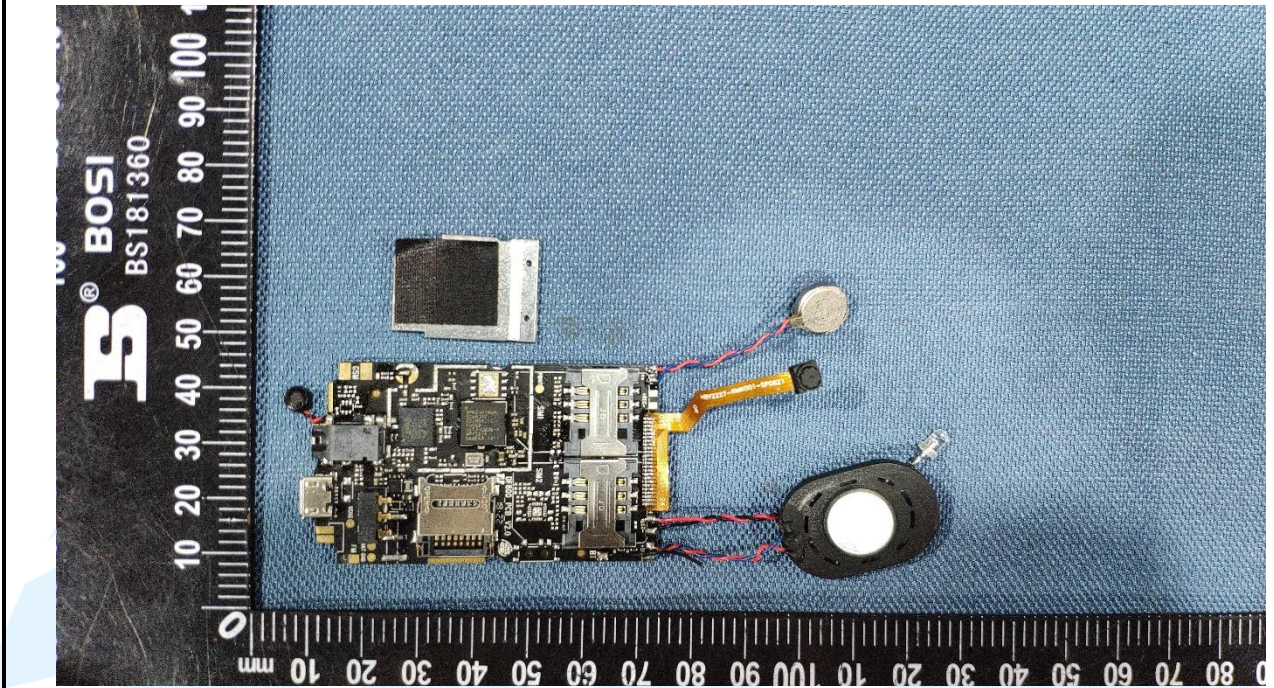
EUT Photo
