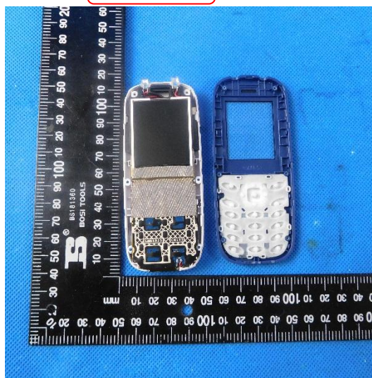
GSM ANT
