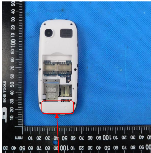
GSM ANT
