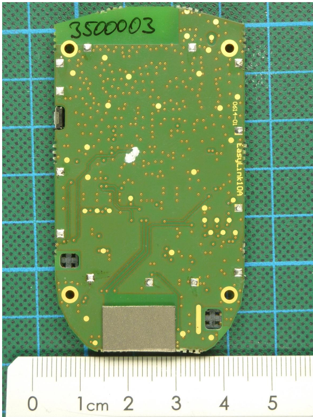
170032_11.JPG: EASYSKAN Link, PCB 2, bottom view
