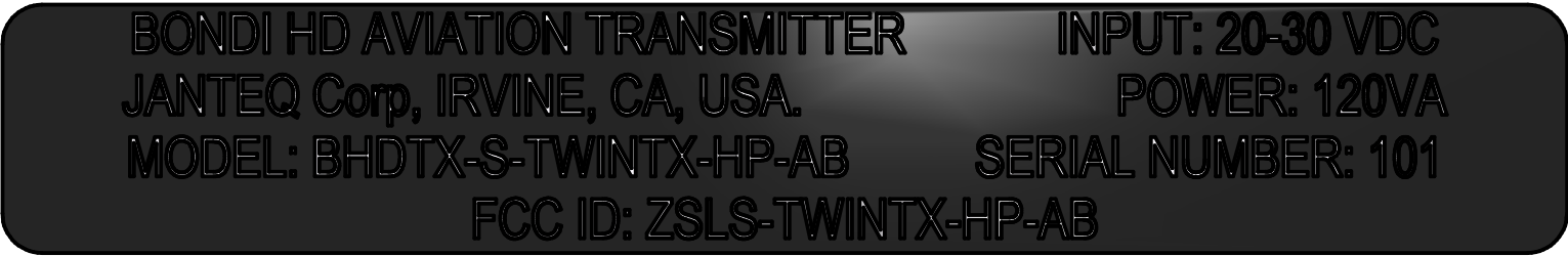
FCC LABEL SCALE 4 : 1
