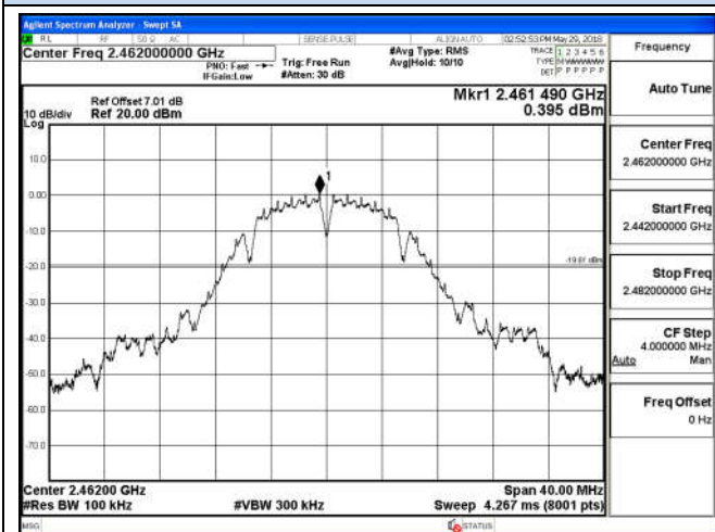
2442 MHz – 2482 MHz
