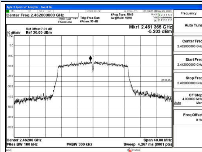
2442 MHz – 2482 MHz
