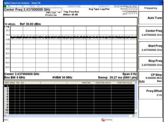
IEEE 802.11g
