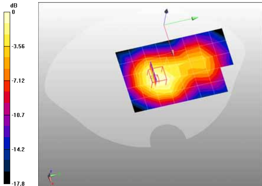
0 dB = 0.109mW/g
