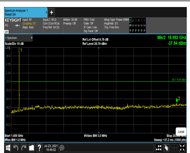
Band2-20MHz-QPSK-18900-1RB#0-Range2:1000~20000MHz
