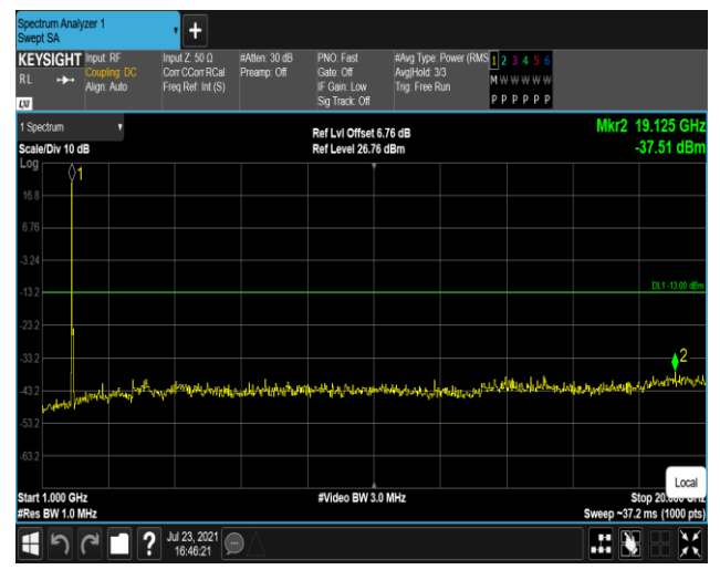
Band2-20MHz-QPSK-19100-1RB#0-Range2:1000~20000MHz
