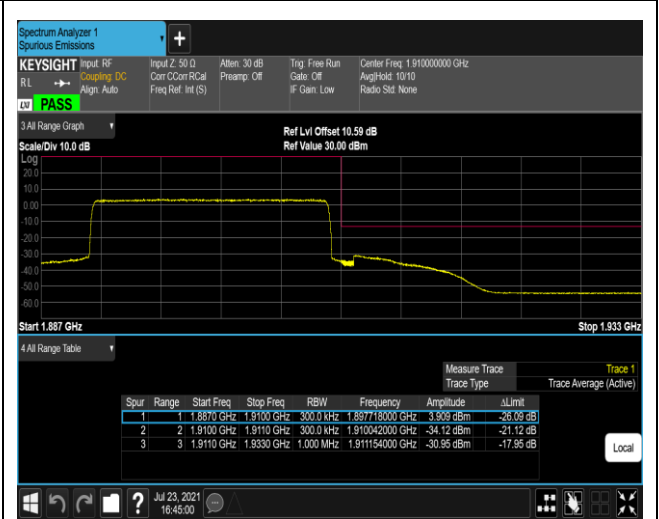
Band2-20MHz-QPSK-19100-100RB#0
