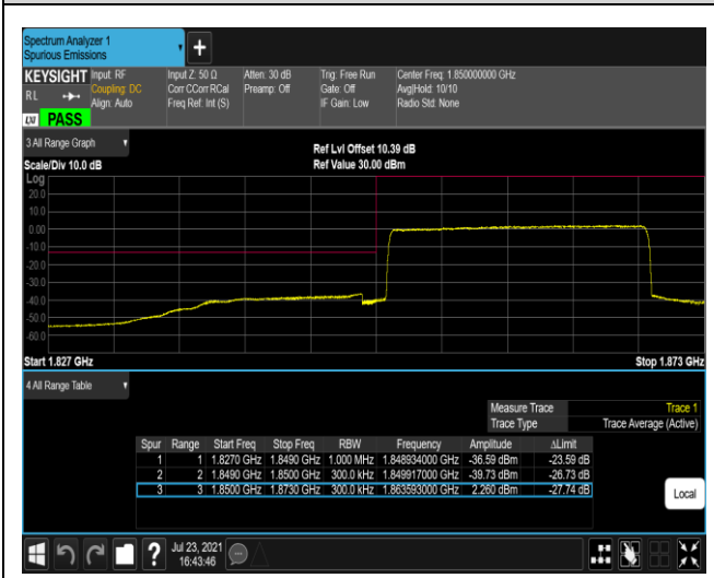
Band2-20MHz-16QAM-18700-100RB#0
