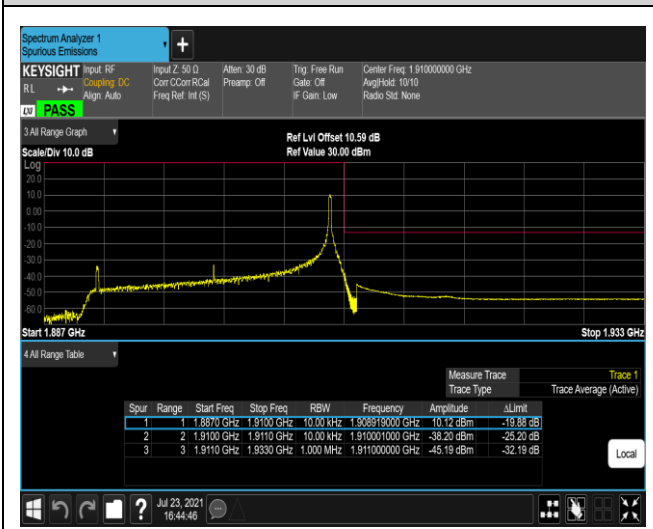
Band2-20MHz-16QAM-19100-1RB#99
