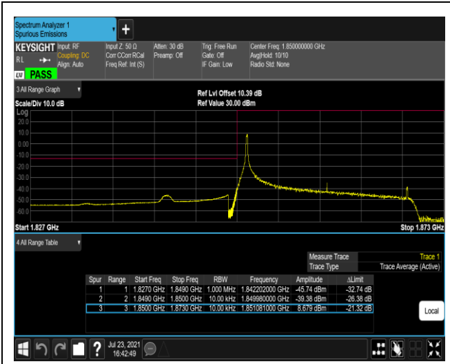
Band2-20MHz-16QAM-18700-1RB#0
