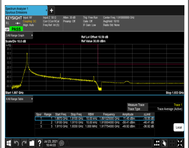
Band2-20MHz-QPSK-19100-1RB#0
