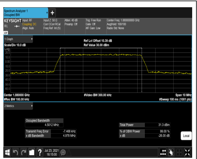
Band2-5MHz-QPSK-18900-25RB#0
