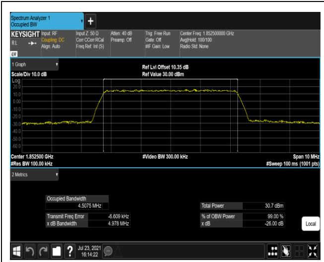
Band2-5MHz-QPSK-18625-25RB#0
