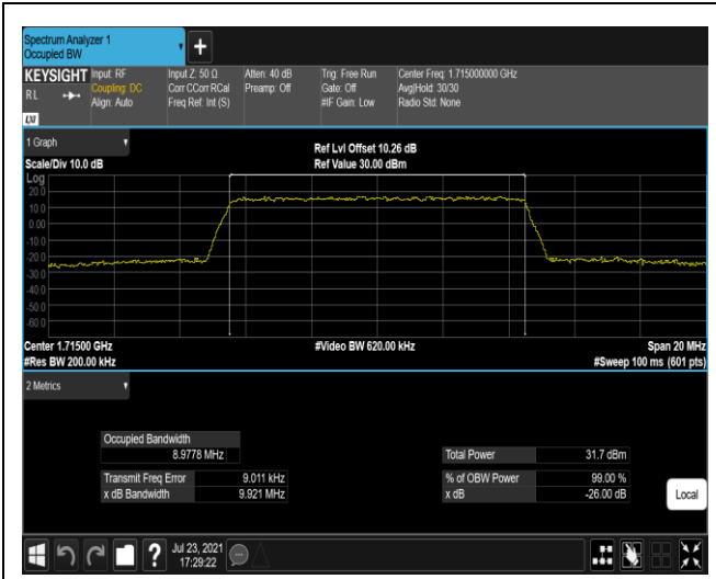
Band4-10MHz-QPSK-20000-50RB#0
