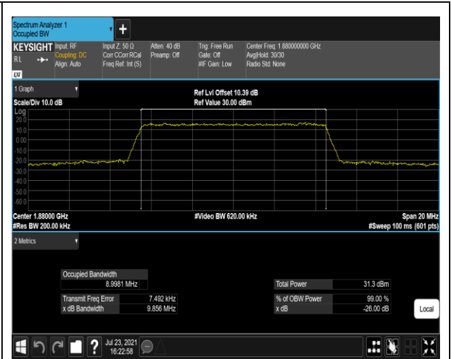
Band2-10MHz-QPSK-18900-50RB#0
