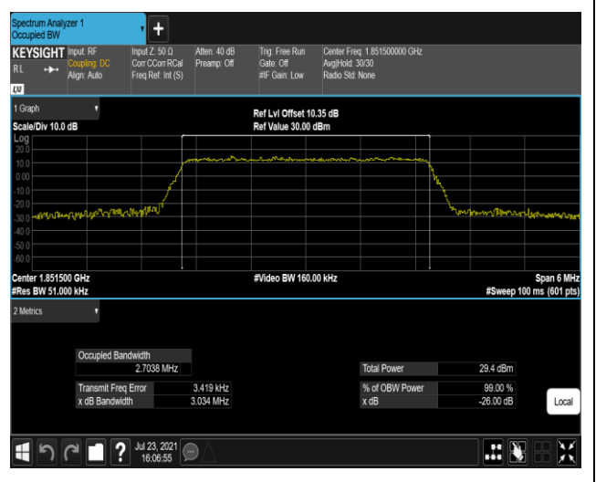
Band2-3MHz-16QAM-18615-15RB#0
