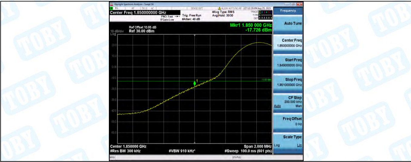
Band2-15MHz-QPSK-18675-1RB#74
