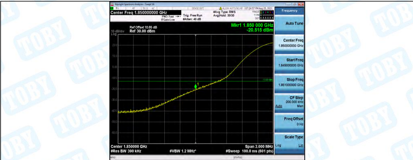
Band2-20MHz-QPSK-18700-1RB#99
