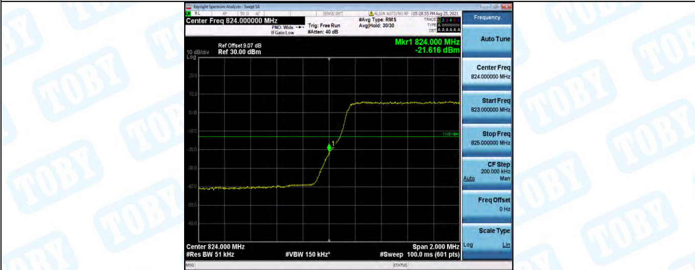
Band5-3MHz-QPSK-20635-15RB#0
