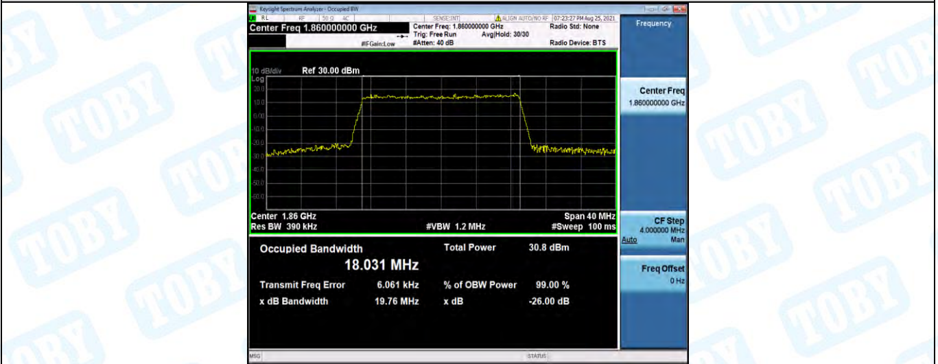
Band2-20MHz-QPSK-18900-100RB#0
