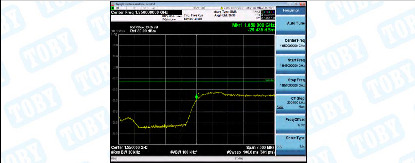
Band2-3MHz-16QAM-18615-15RB#0
