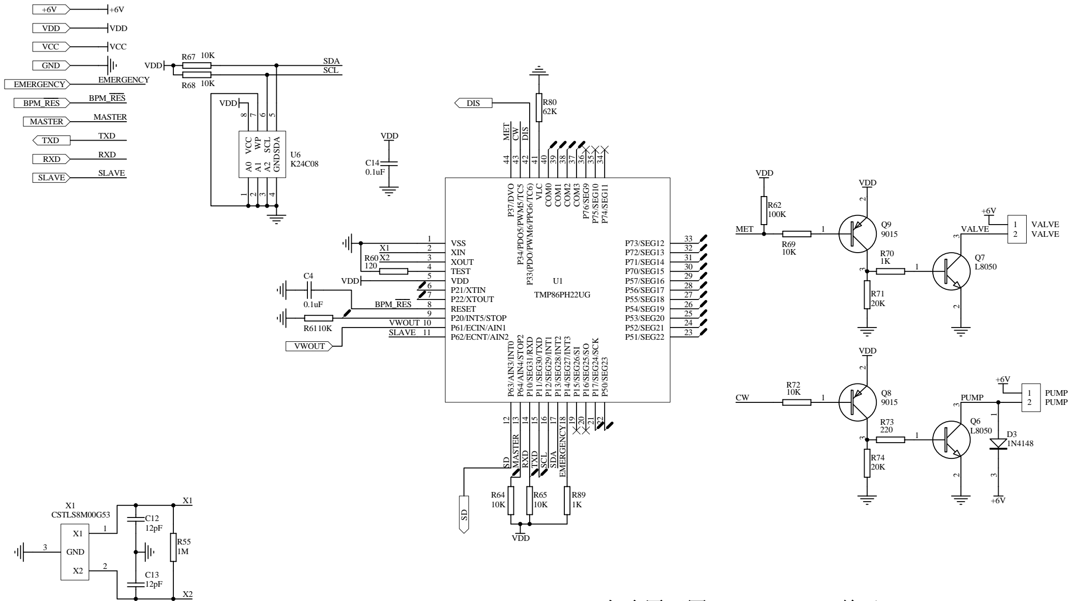
KD-923 电路原理图—MCU_BPM 单元
