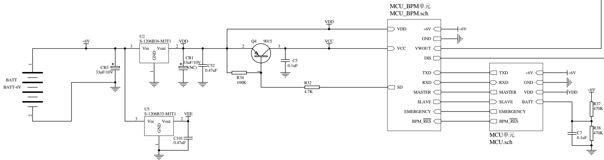
KD-923 电路原理图—电源、放大单元
