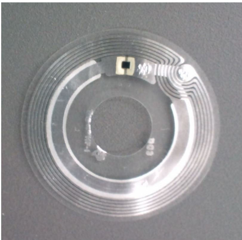
IC_Tag(Rear side)
